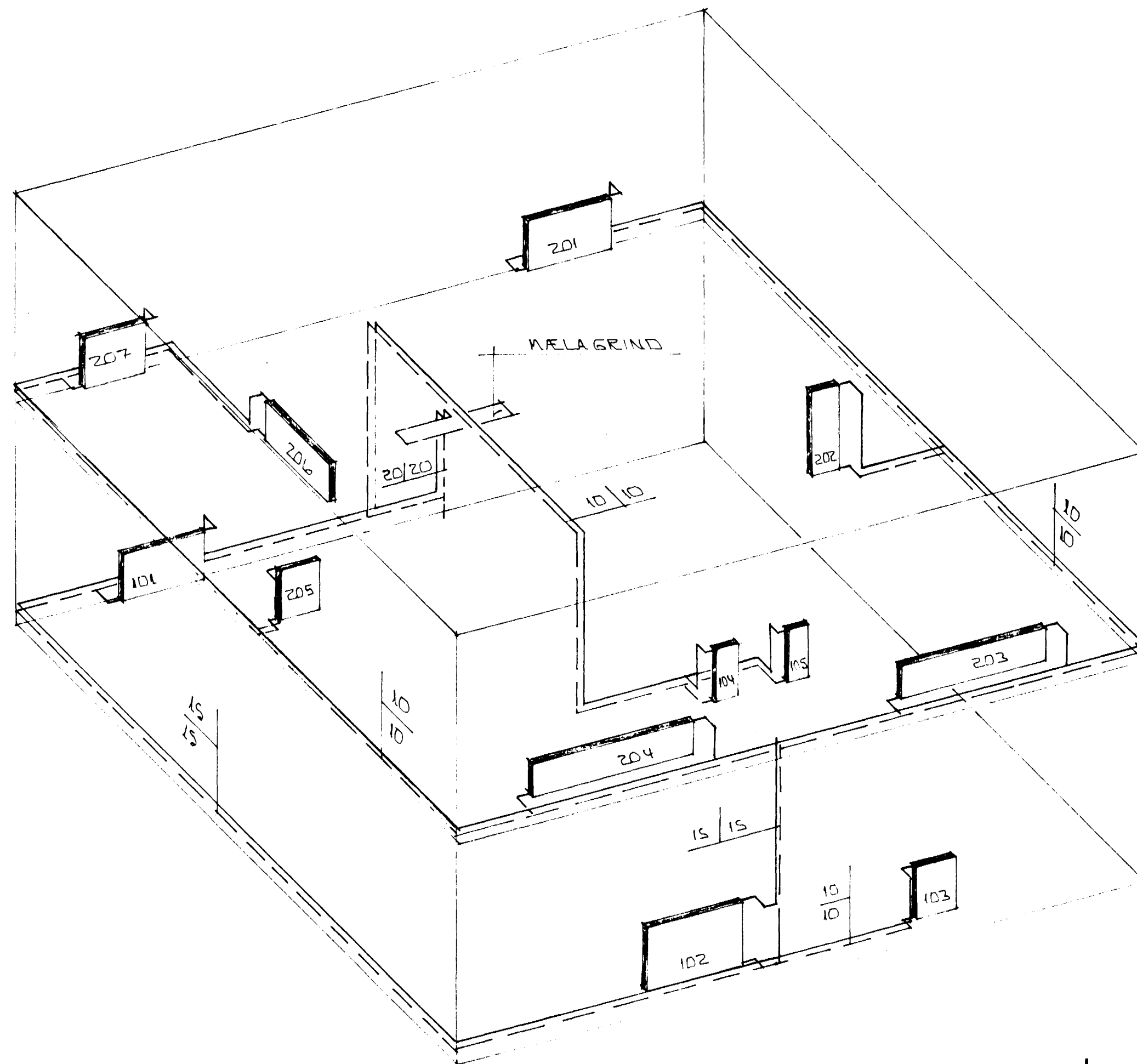
RÚMMYND HITALAGNA 1:50
