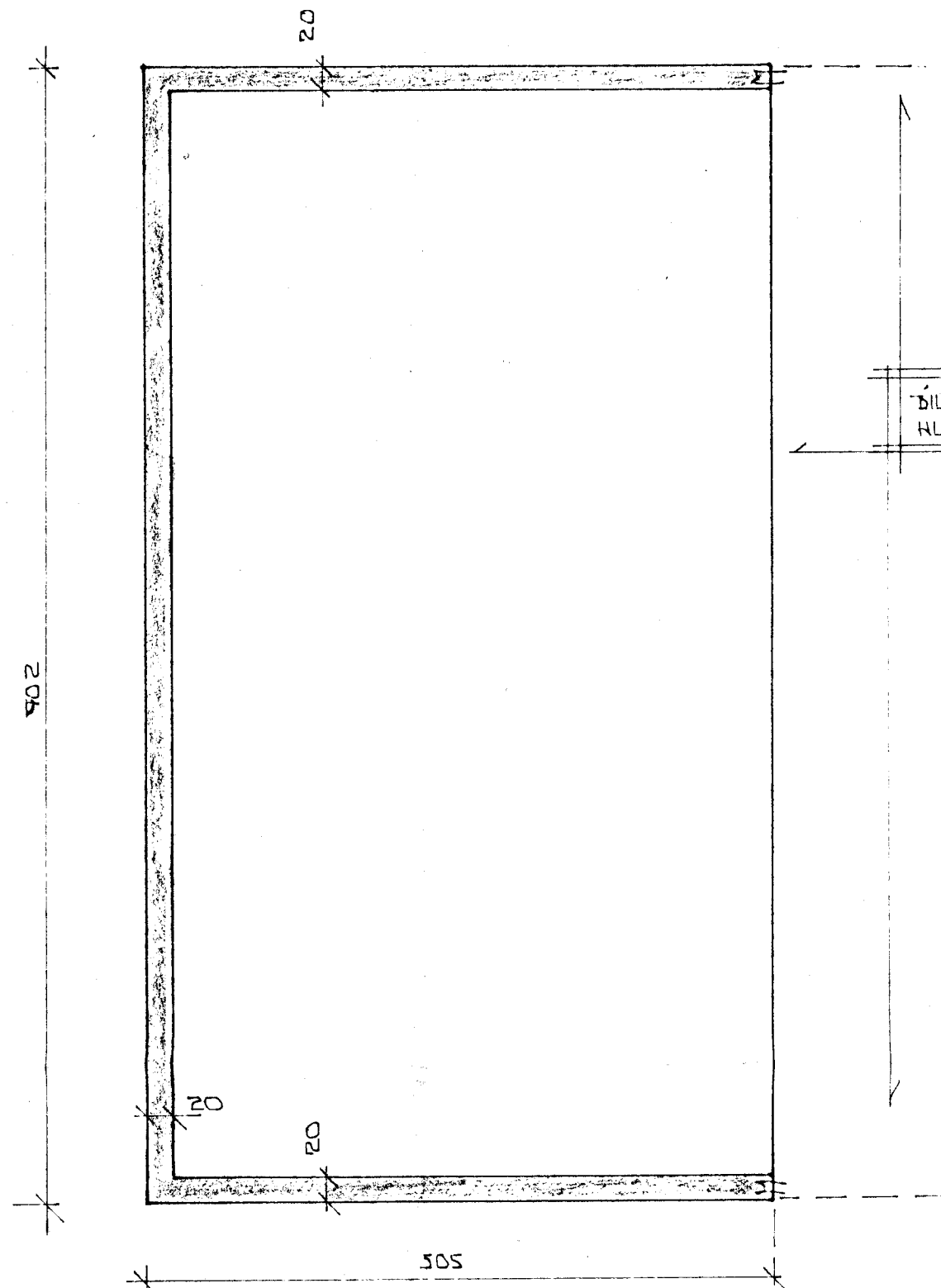
GRUNNMYND UNDIRSTÖÐUR 1:50
