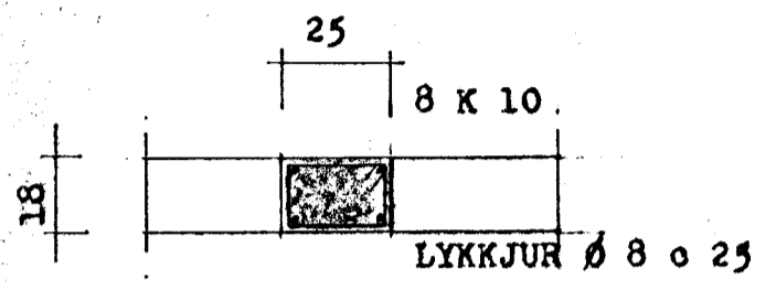
SÓLA S - 1 1:20
