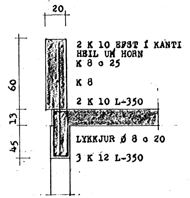
SNID - B 1:20
