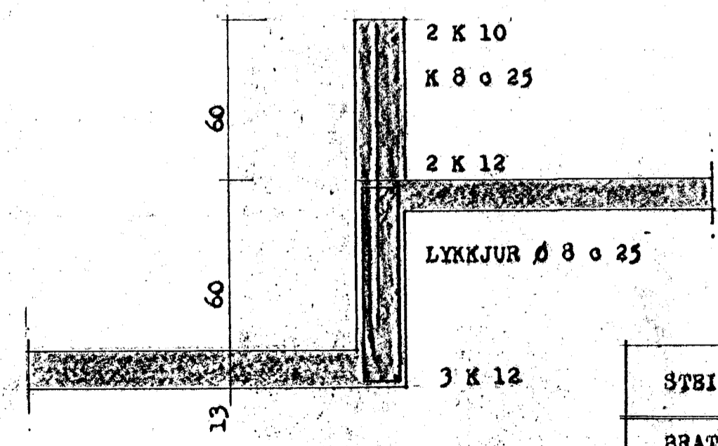
SNID - D 1:20
