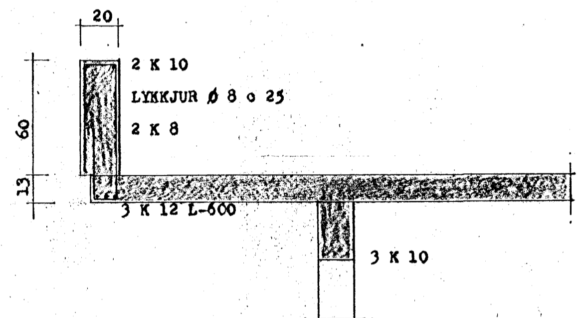
SNID - C 1:20
