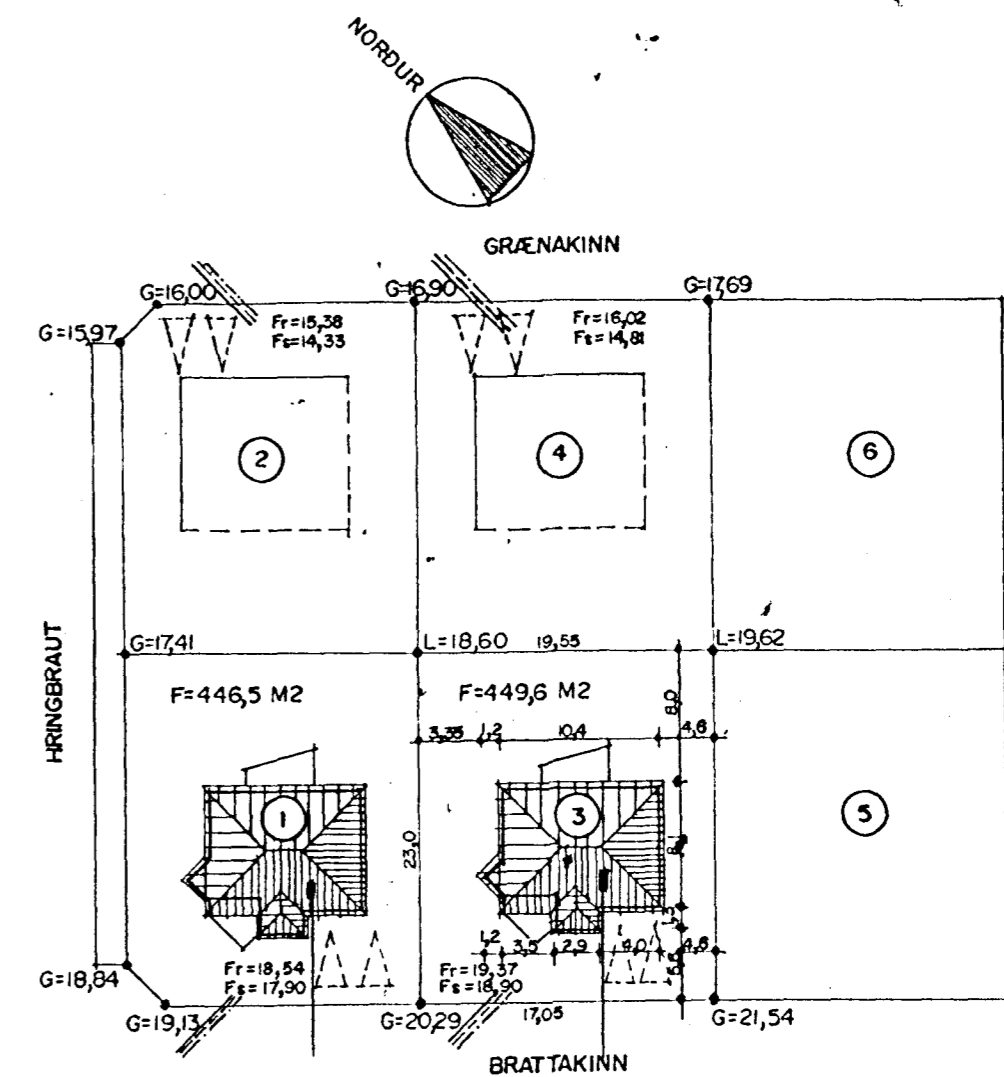
AFSTÖÐUMYND MKV. 1:500
