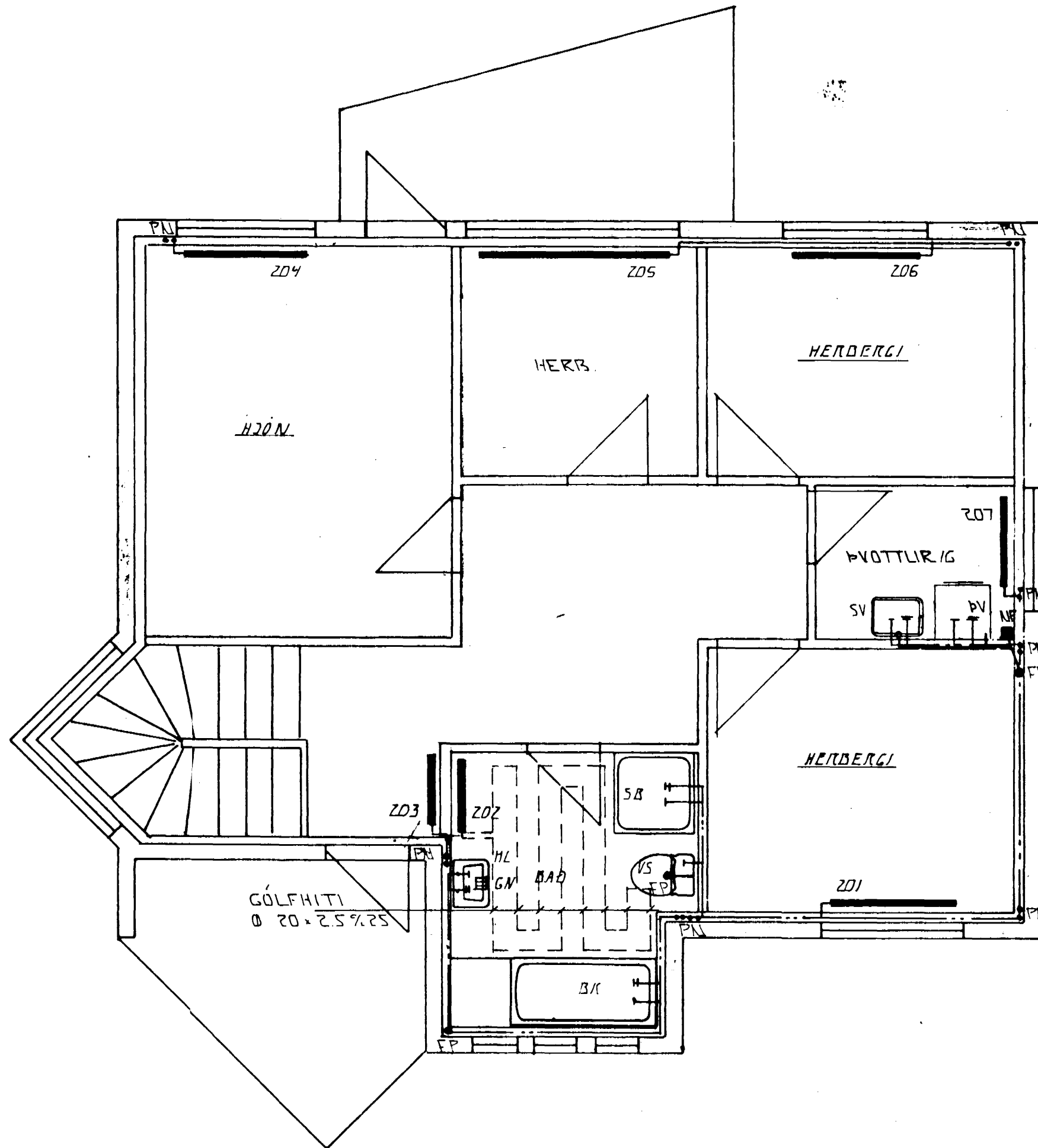
GRUNNMÝND . 2. HÆÐ . 1:50
