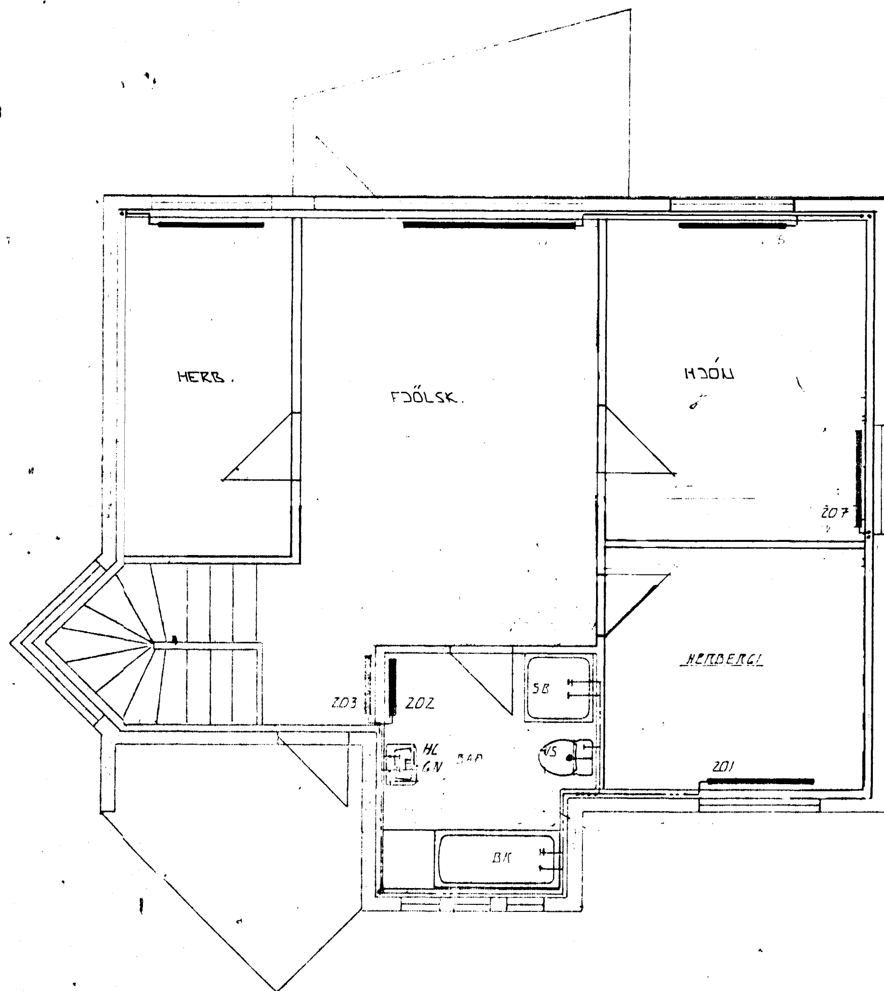
GRUNNMUND . 2. HÆÐ . 1:50
