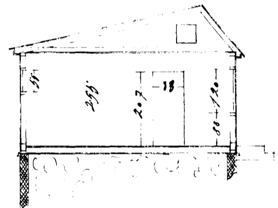
Þverskurður
