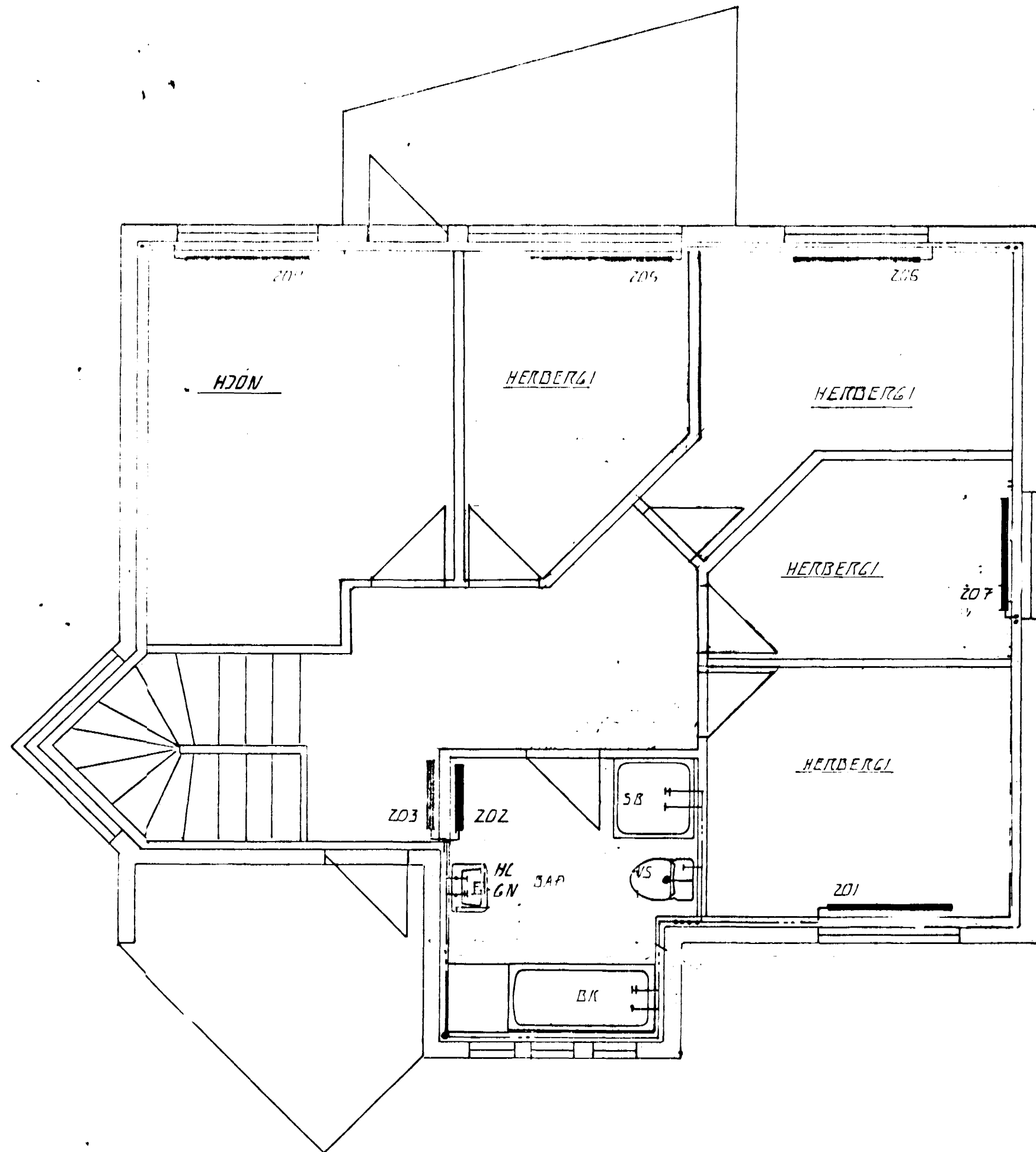
GRUNNMUND . 2. HÆÐ . 1:50
