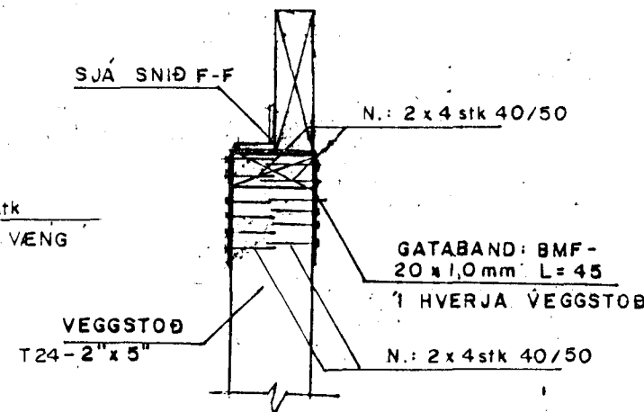
SNID B-B M. 1:10
