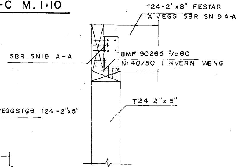
SNID F-F M. 1:10
