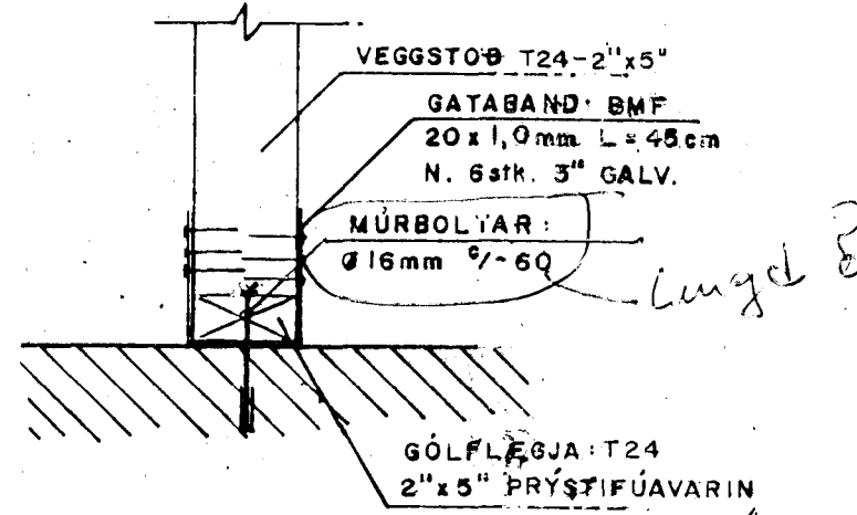
SNID D-D M. 1:10
