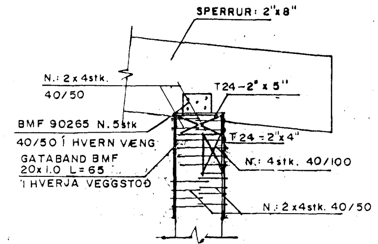
SNID C-C M. 1:10
