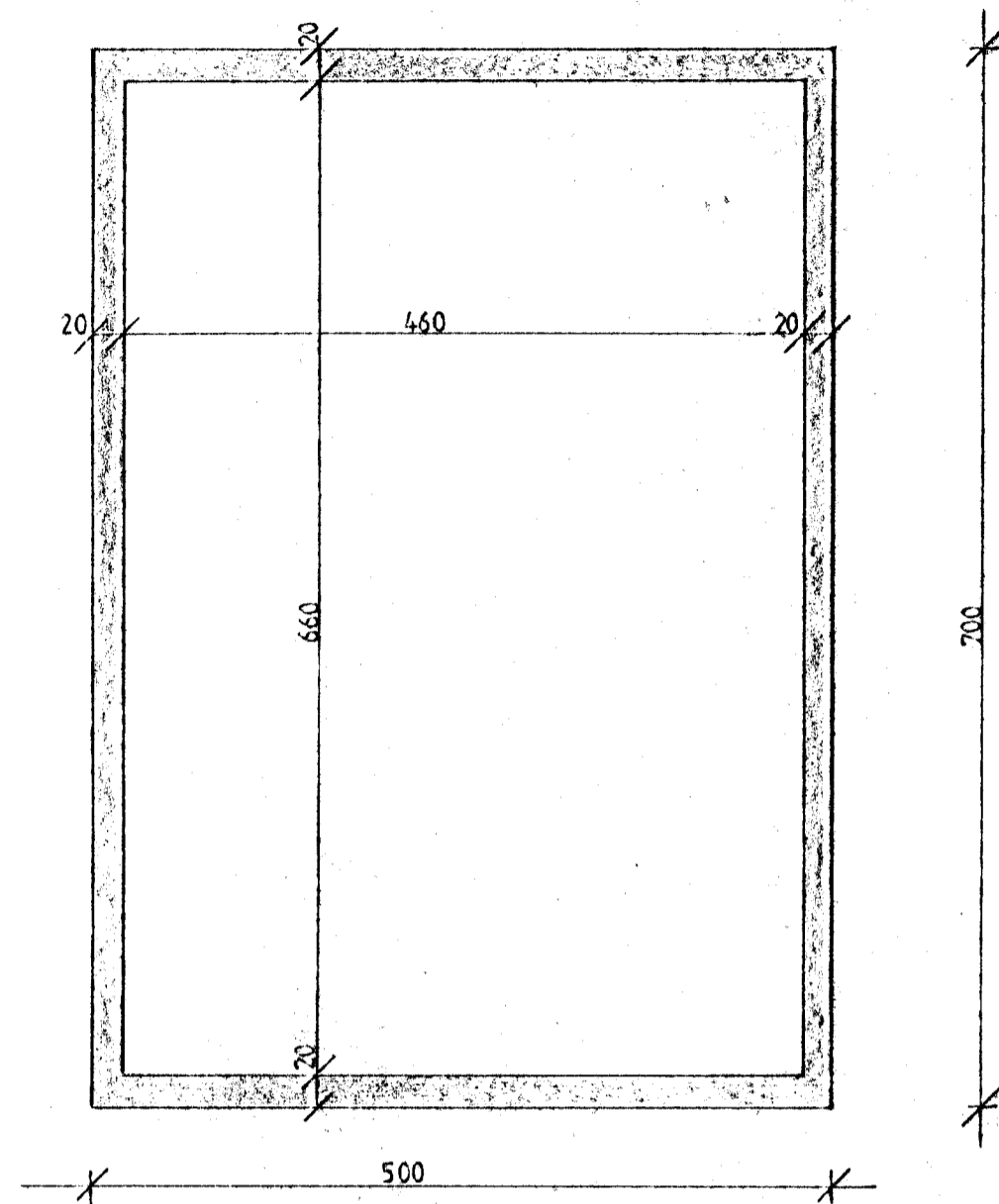
UNDIRSTÖÐUR 1:500
