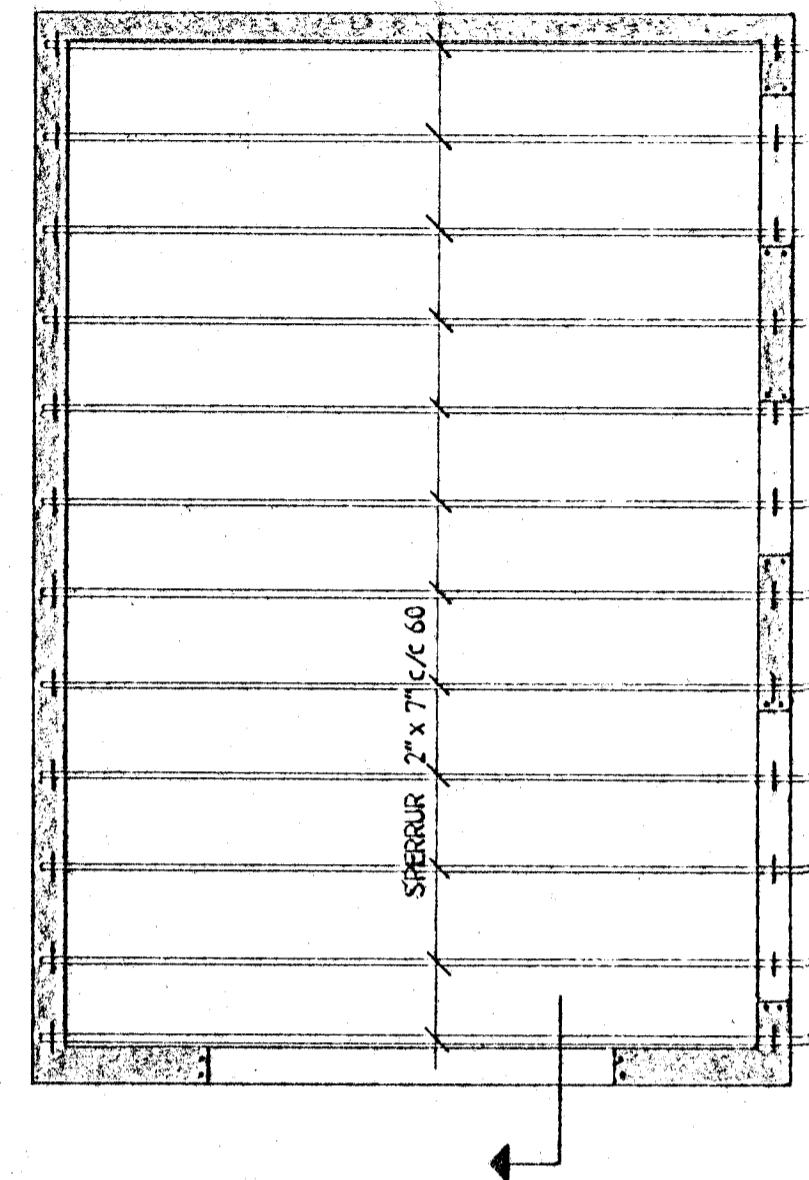
ÞAK 1:500
