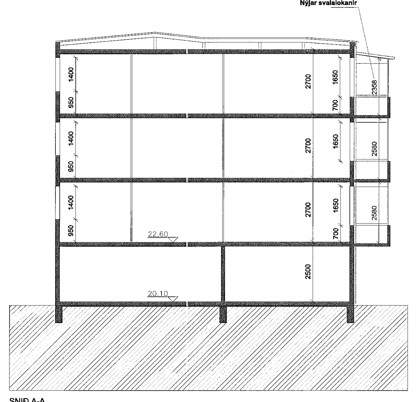
SNID A-A
