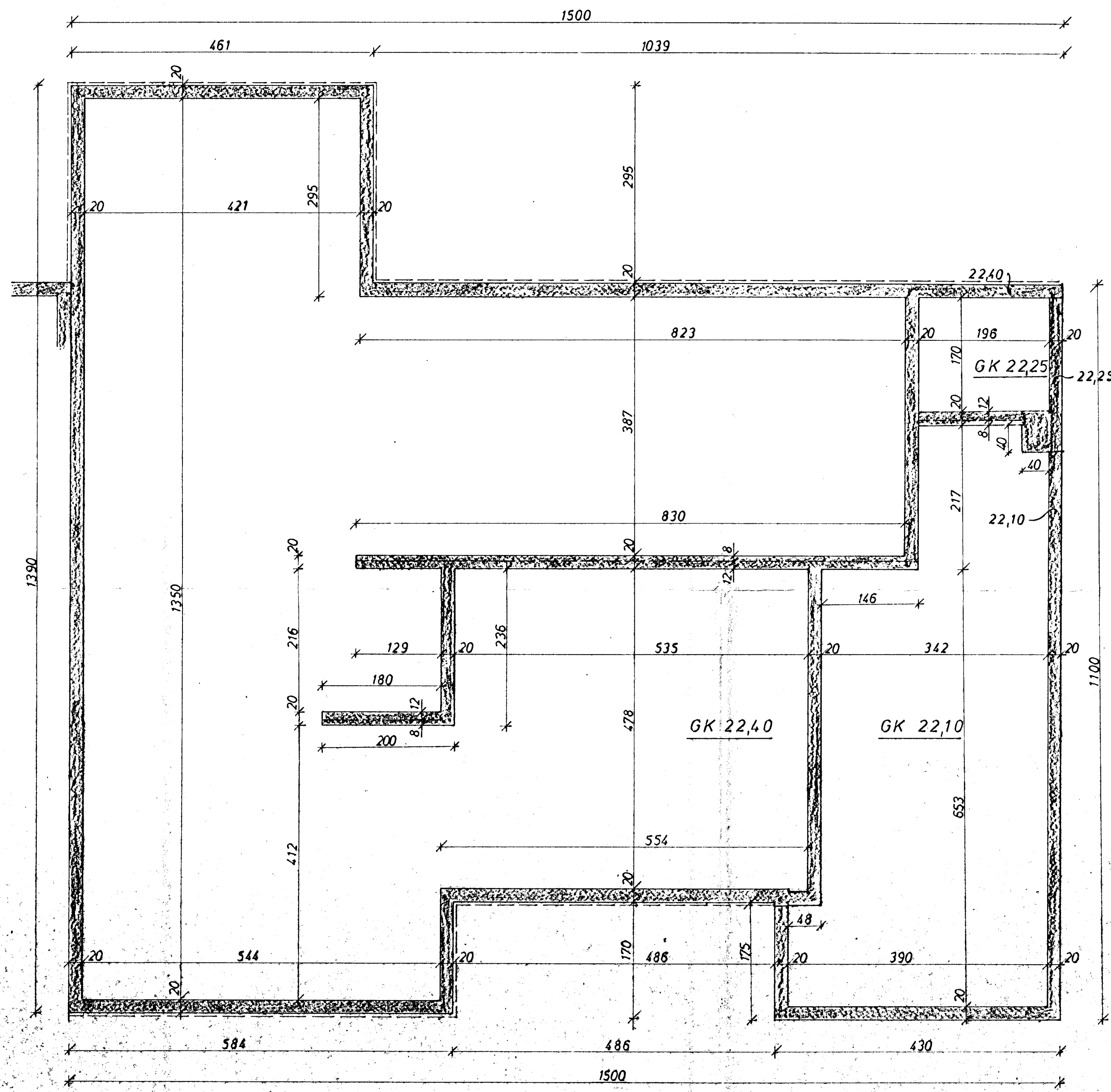
GRUNNMYND 1:50
