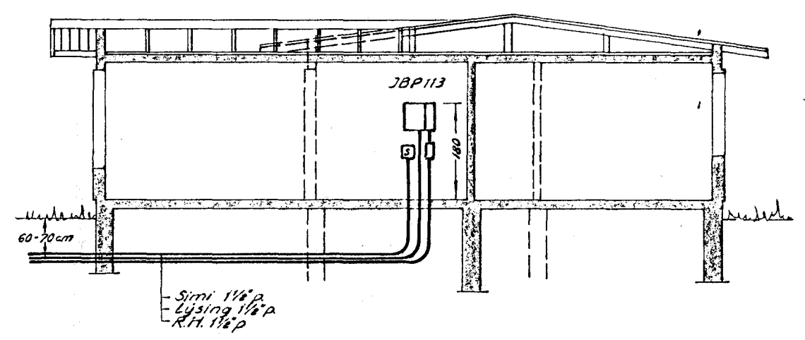
ÞVERSNID B-B M=1:100
