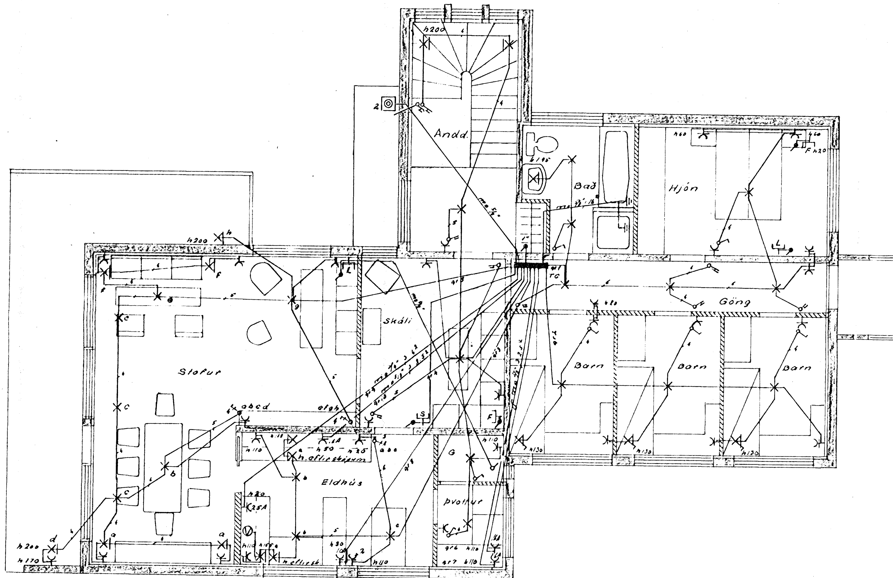
Grunnmynd 2. hæðar
