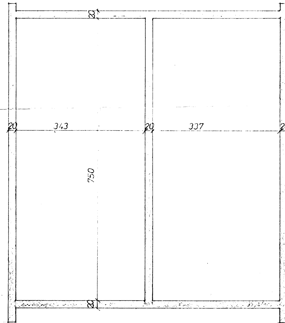
UNDIRSTÖÐUR
