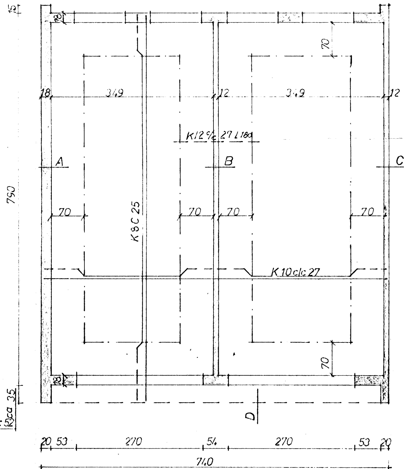
LOFTPLATA BILGEYMSLU
