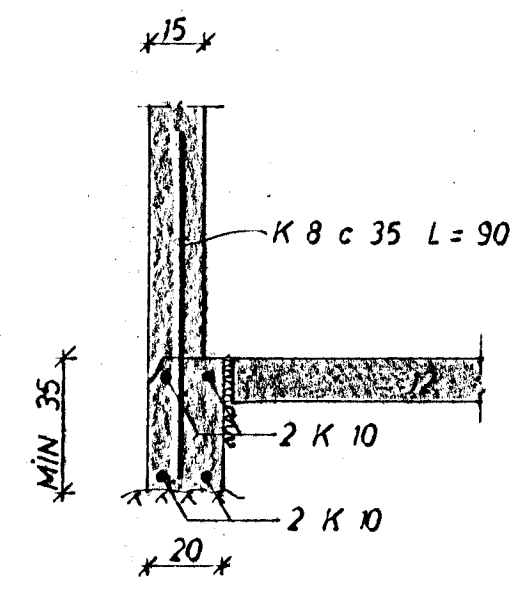
SNID I UTVEGG 1:20
