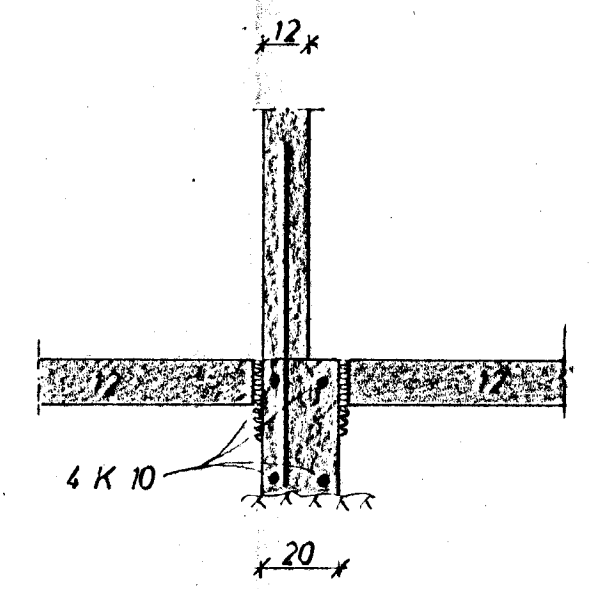
SNID I INNVEGG 1:20
