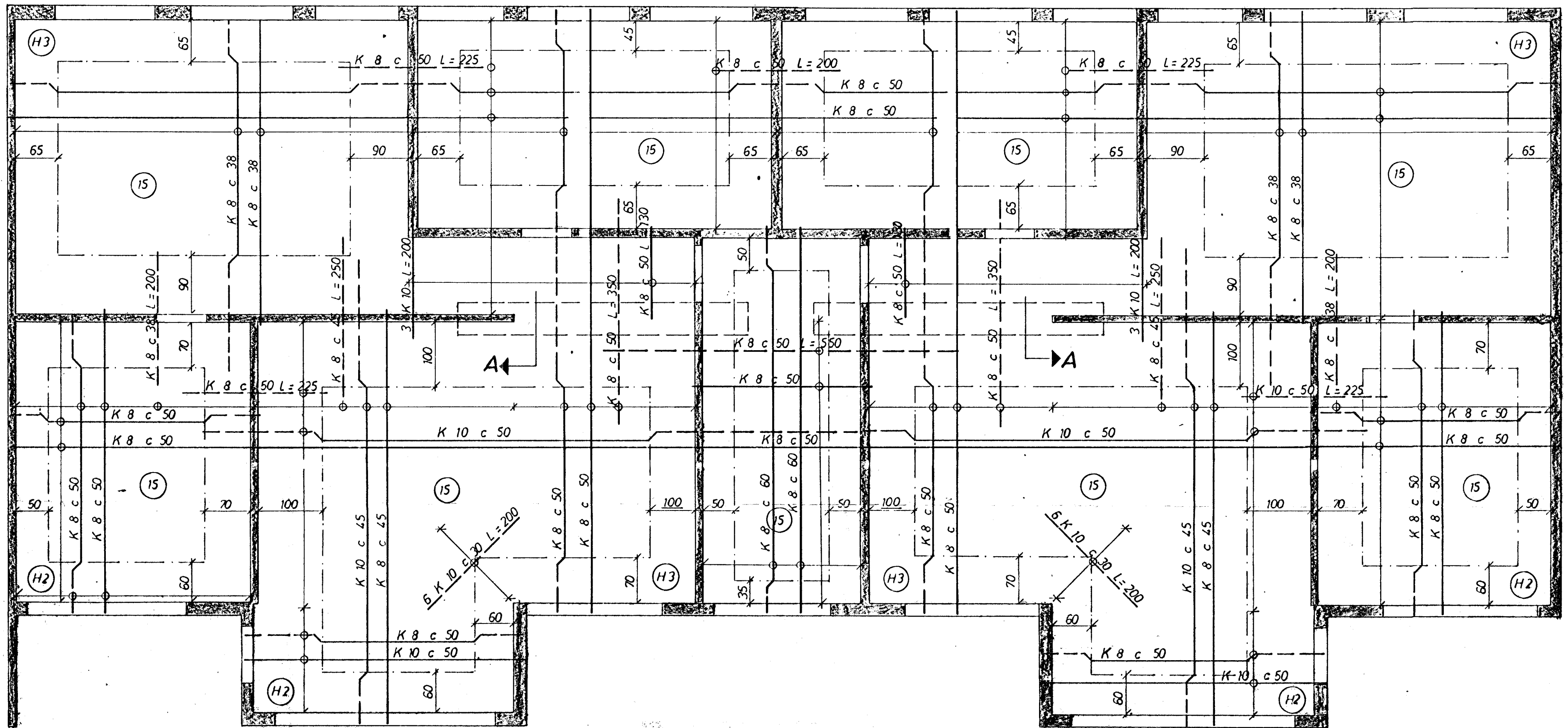
GRUNNMYND 1:50
