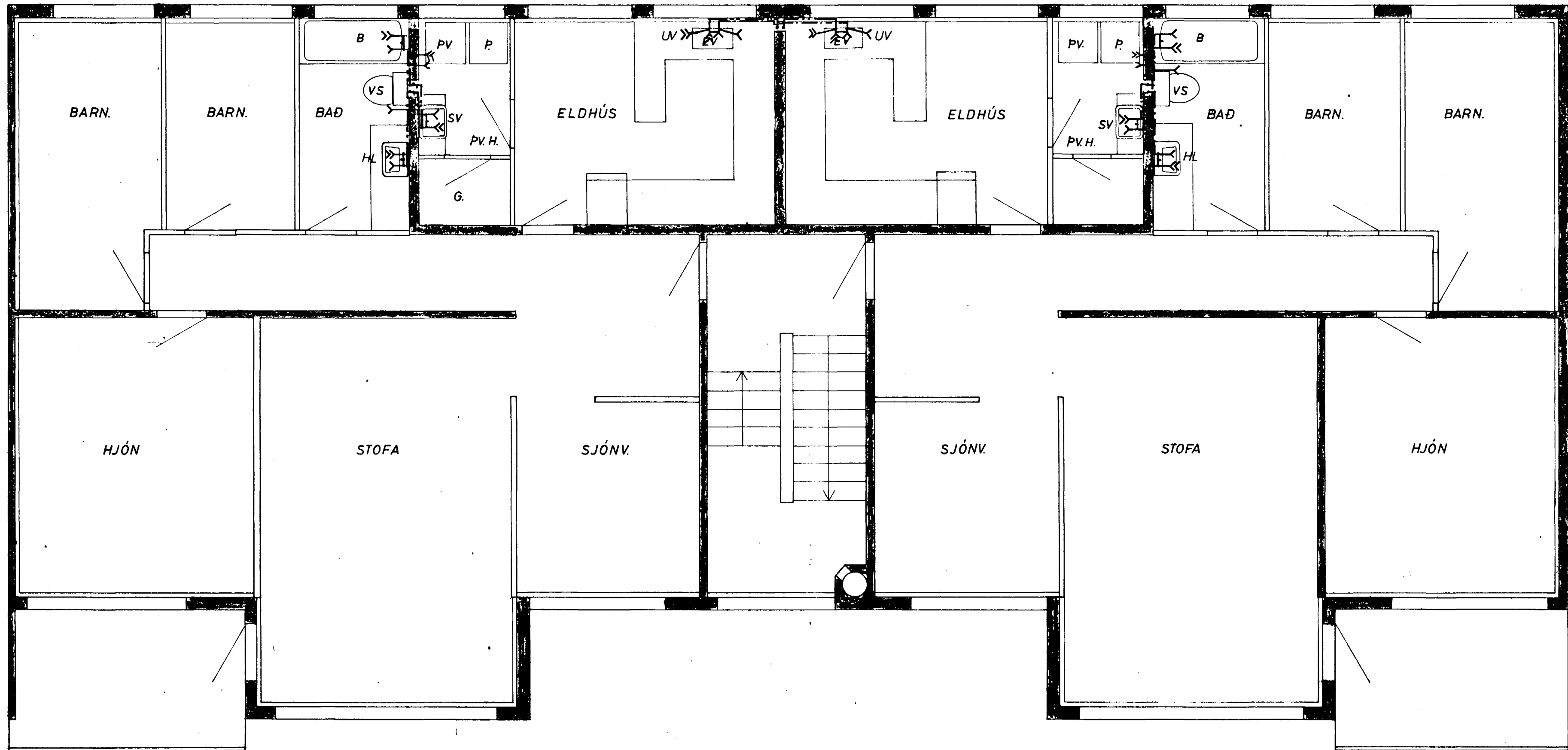
GRUNNMYND MKV. 1:50
