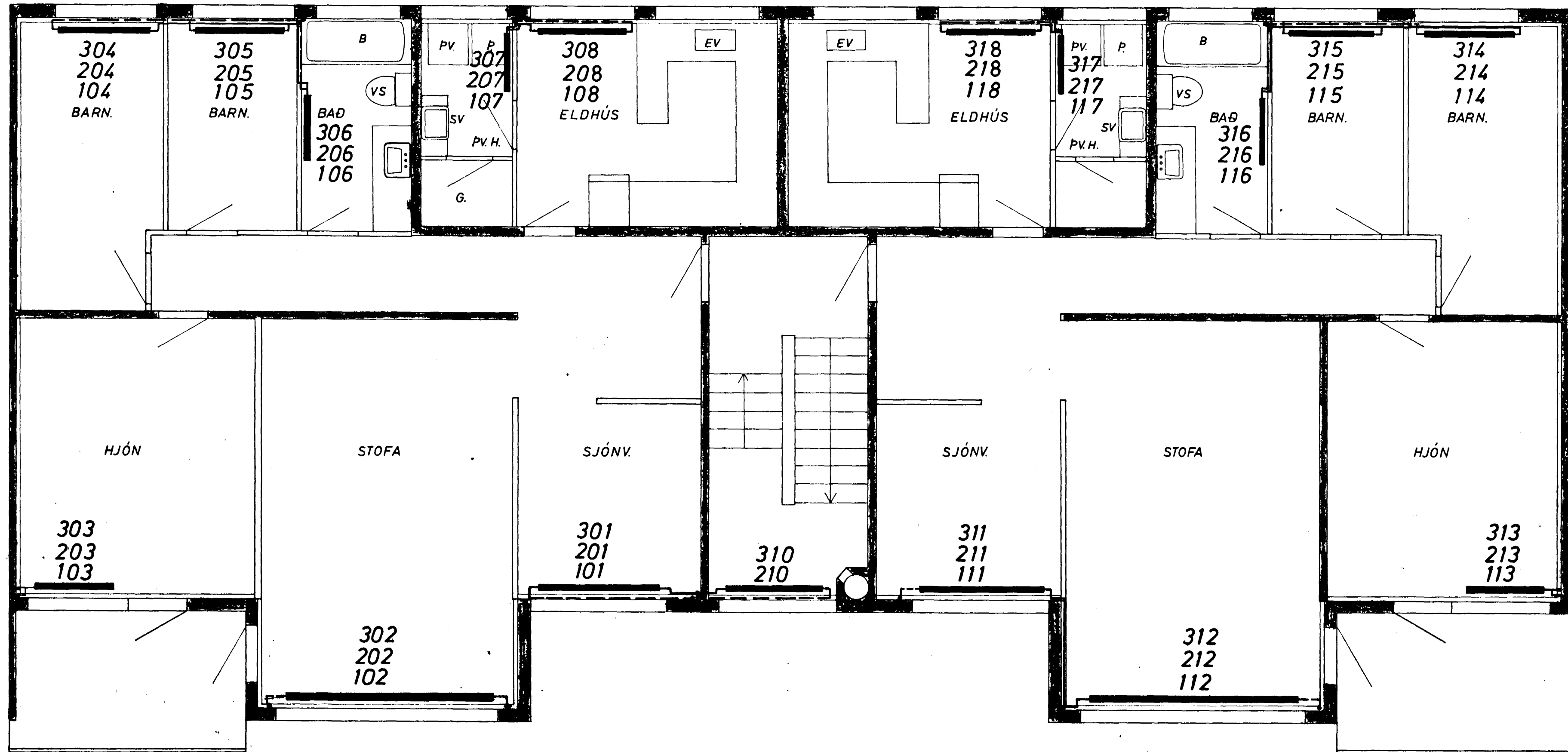
GRUNNMYND MKV. 1:50
