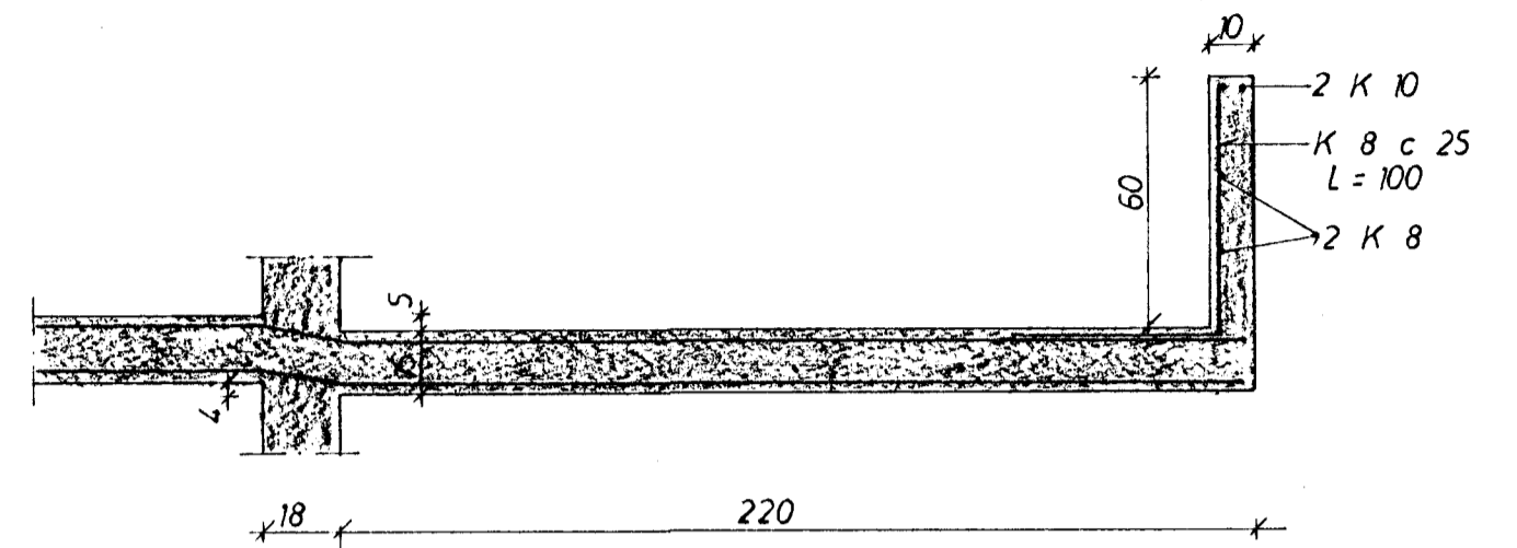
SNID '1 ALLAR SVALIR 1:20
