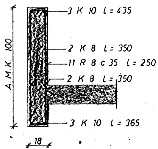
1. OG 2. HÆÐ
