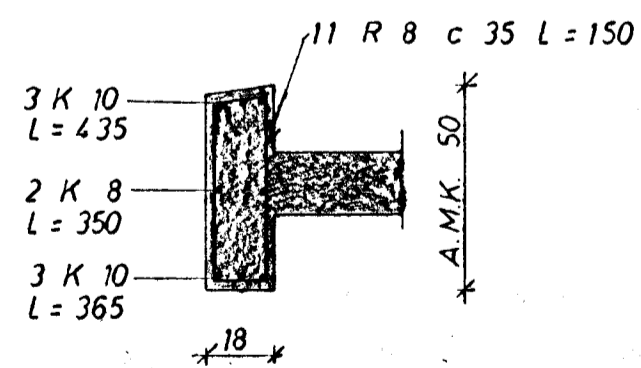
3. HÆÐ
