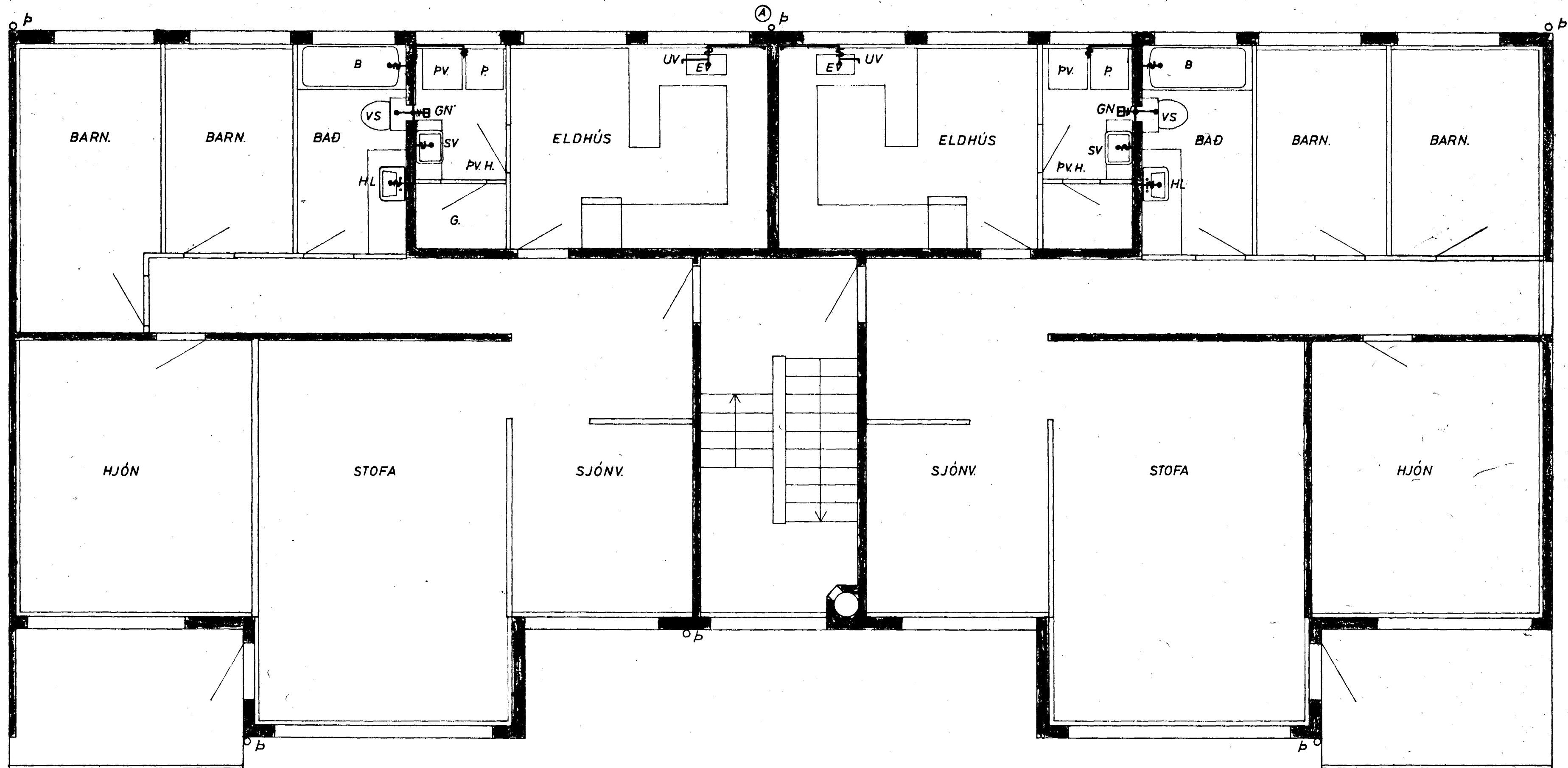
GRUNNMYND MKV. 1:50
