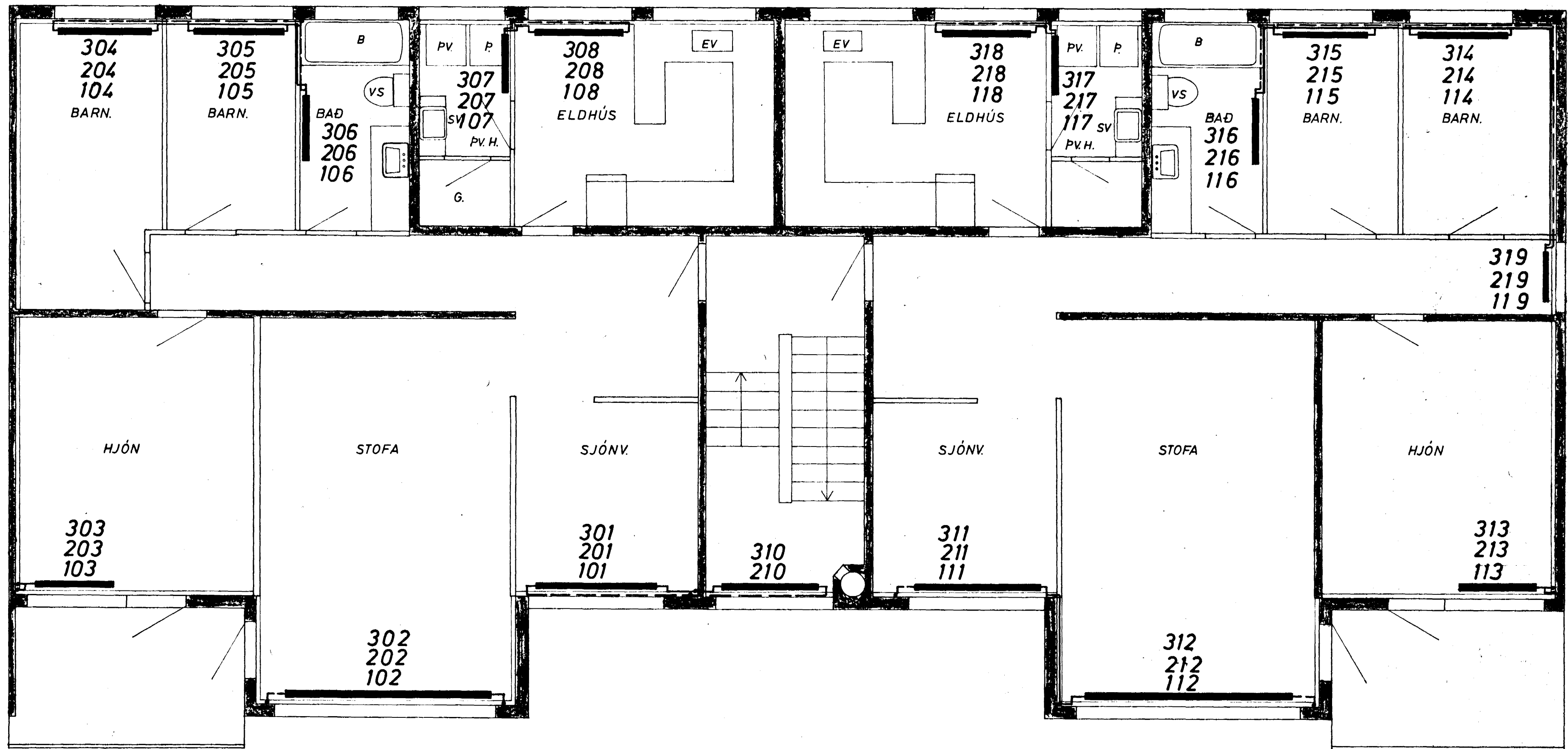
GRUNNMYND MKV. 1:50
