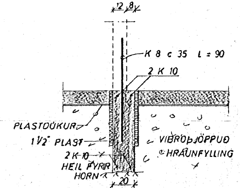
SNID 1 INNVEGG 1:20
