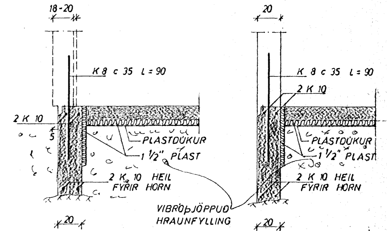
SNID 1 ÚTVEGGI 1:20
