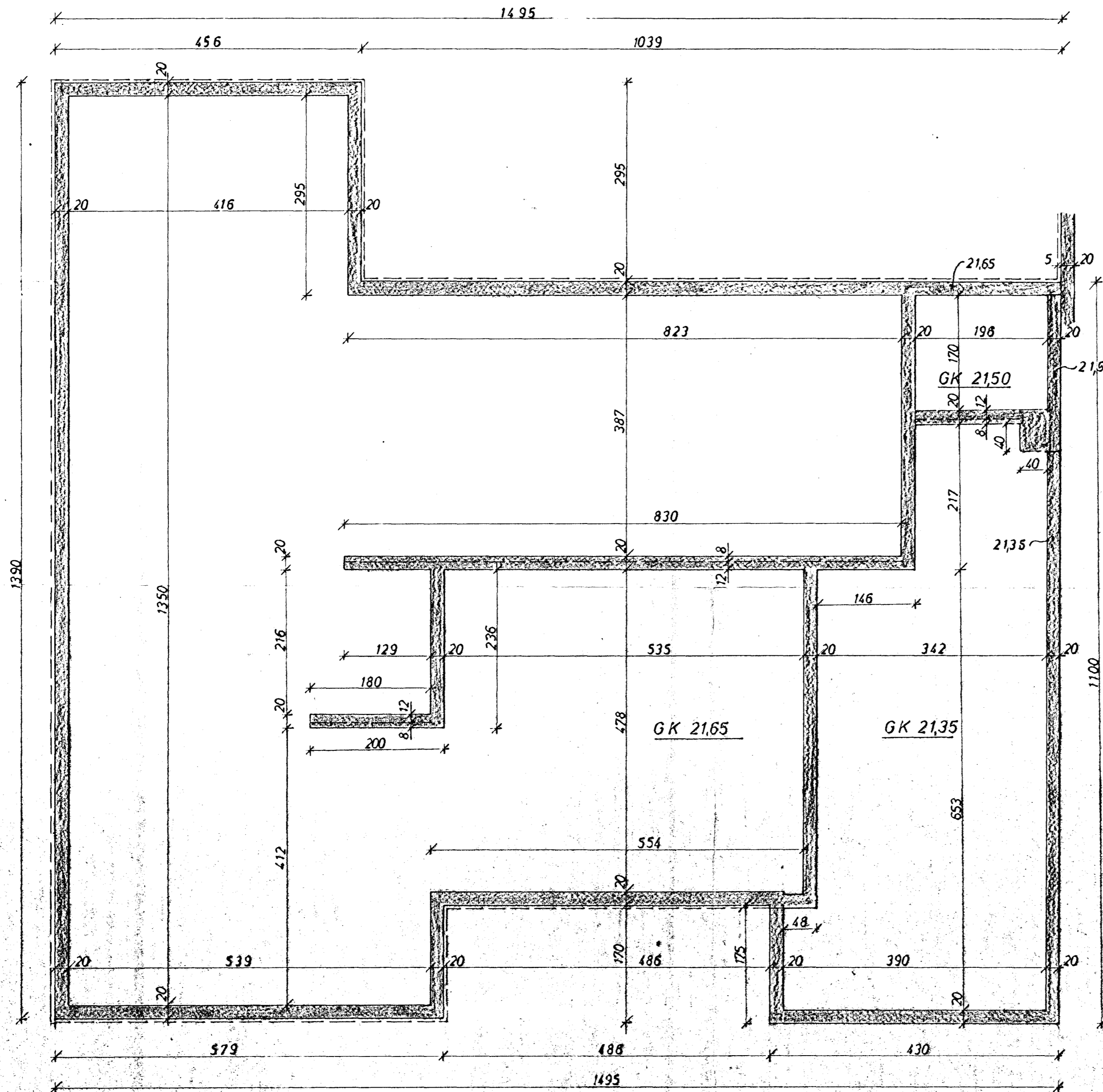
GRUNNMYND 1:50
