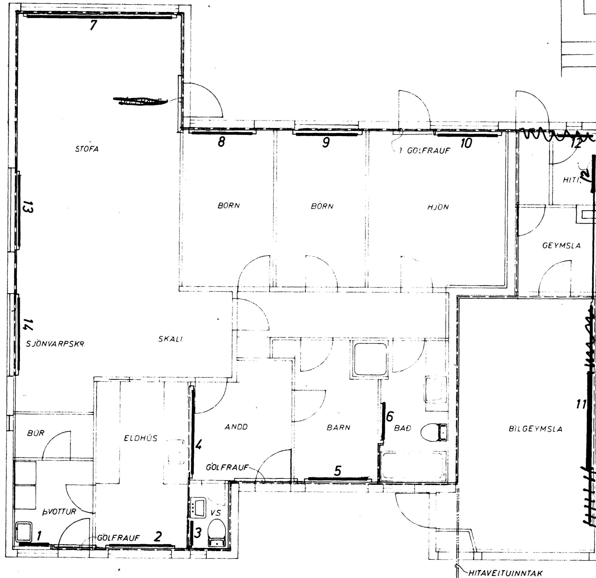
GRUNNMYND 1:50
