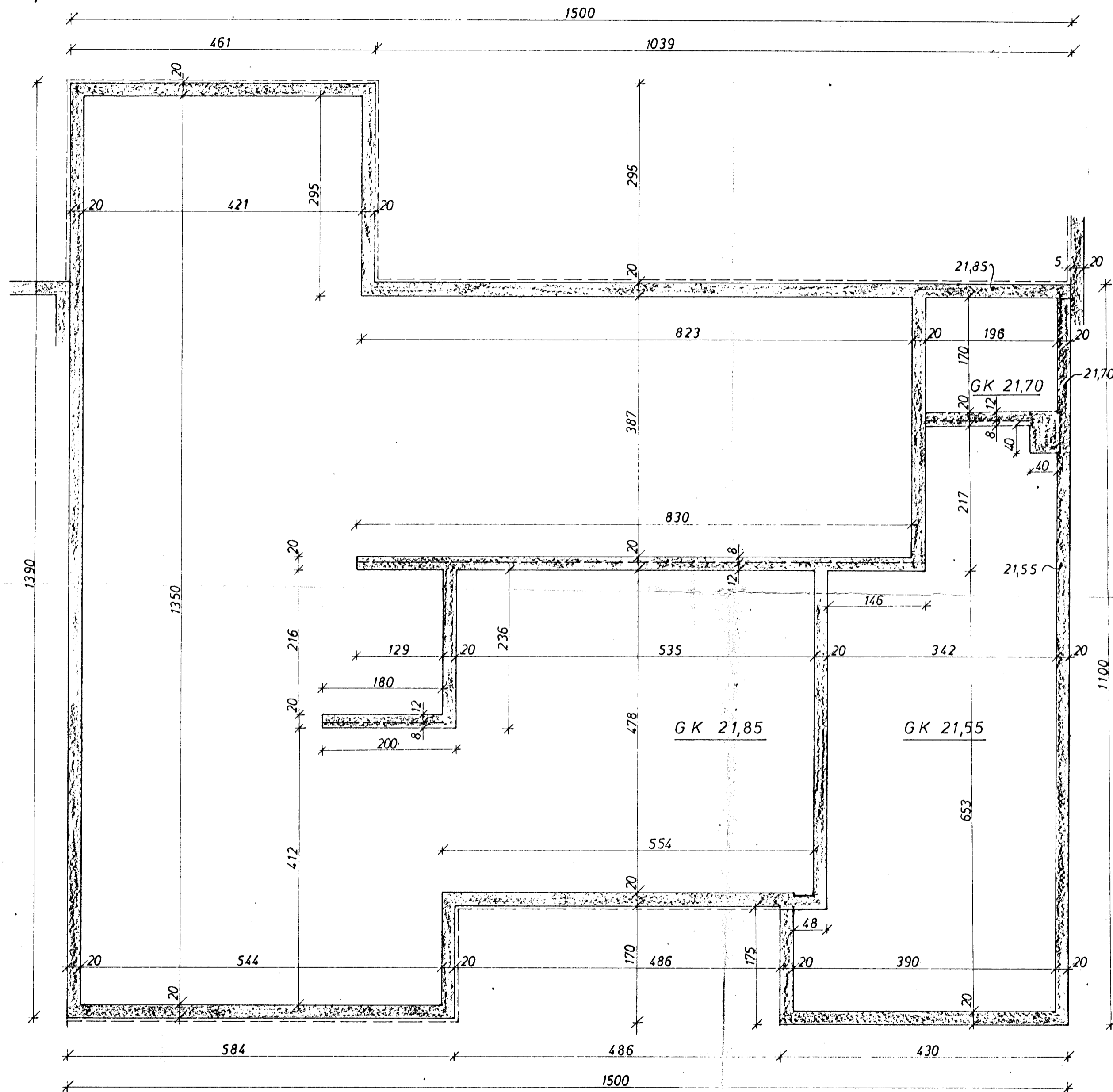
GRUNNMYND 1:50
