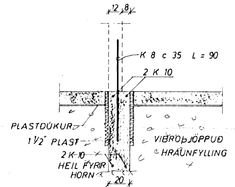
SNID 1 INNVEGG 1:20
