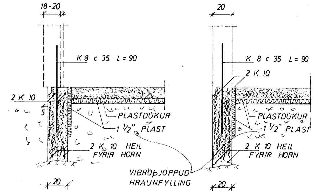
SNID 1 ÚTVEGGI 1:20
