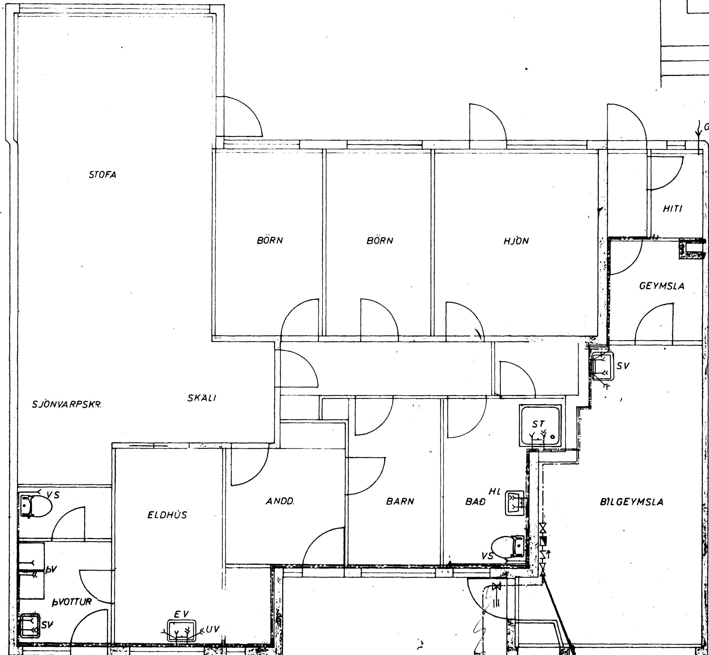
GRUNNMYND 1:50
