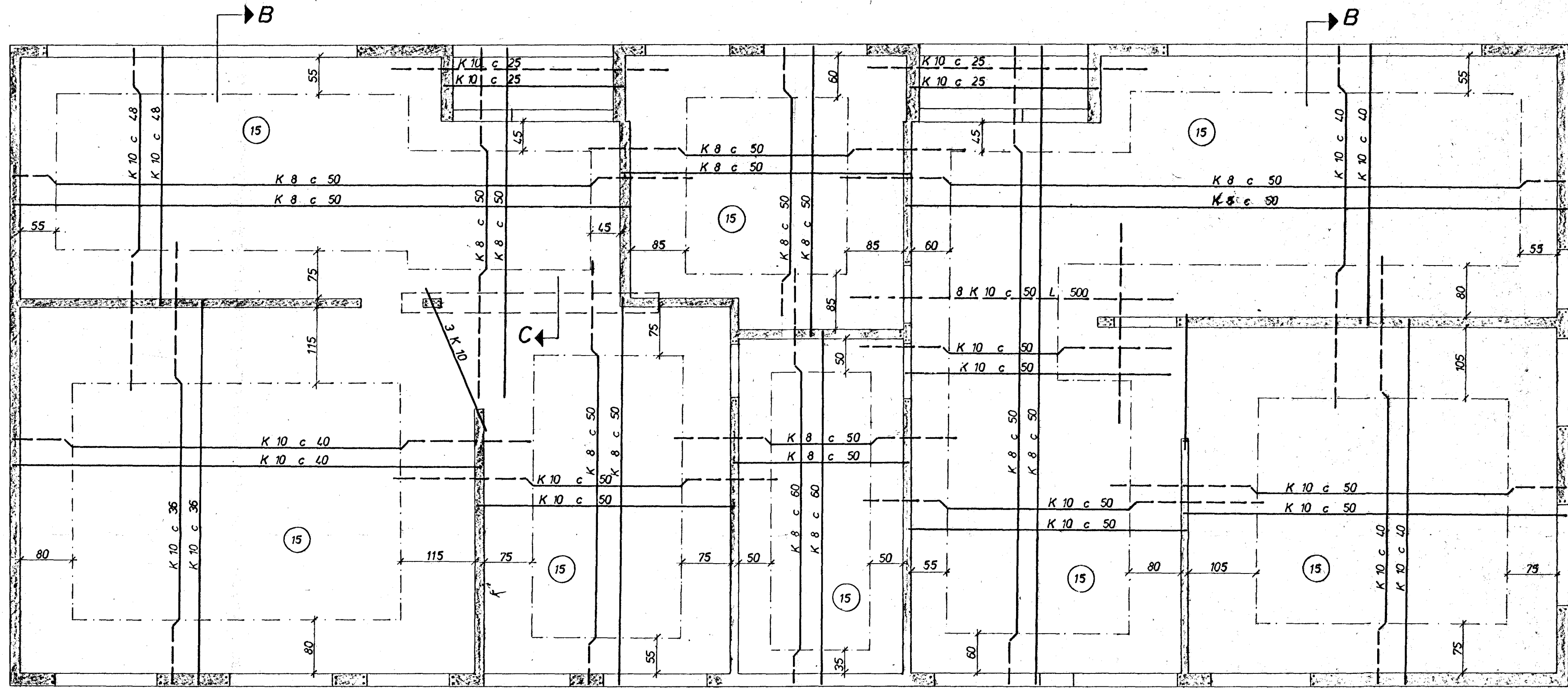
GRUNNMYND 1:50
