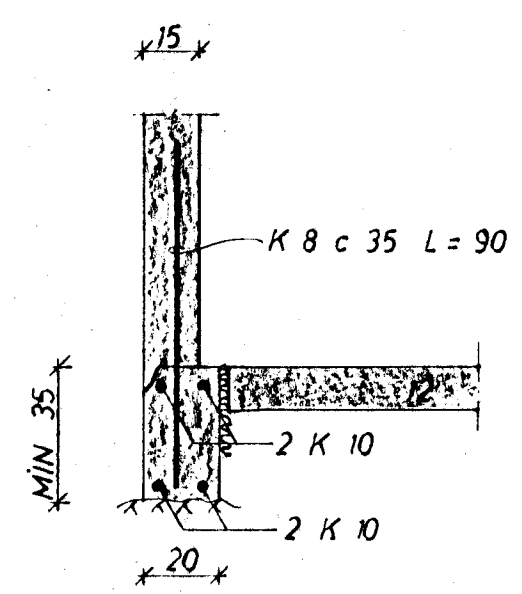
SNID '1 ÚTVEGG 1:20
