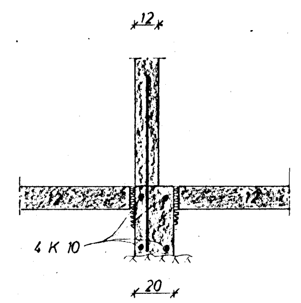
SNID '1 INNVEGG 1:20
