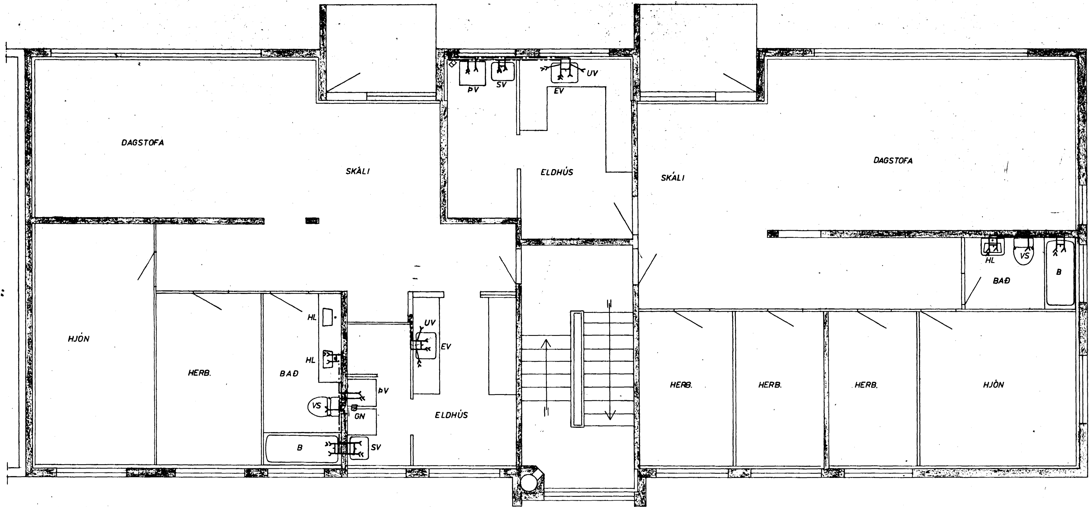
GRUNNMYND 1:50
