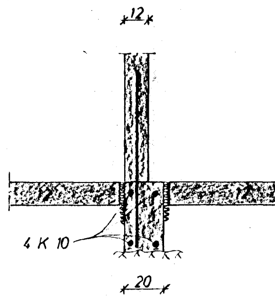
SNID '1 INNVEGG 1:20
