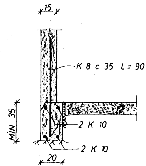
SNID '1 ÚTVEGG 1:20
