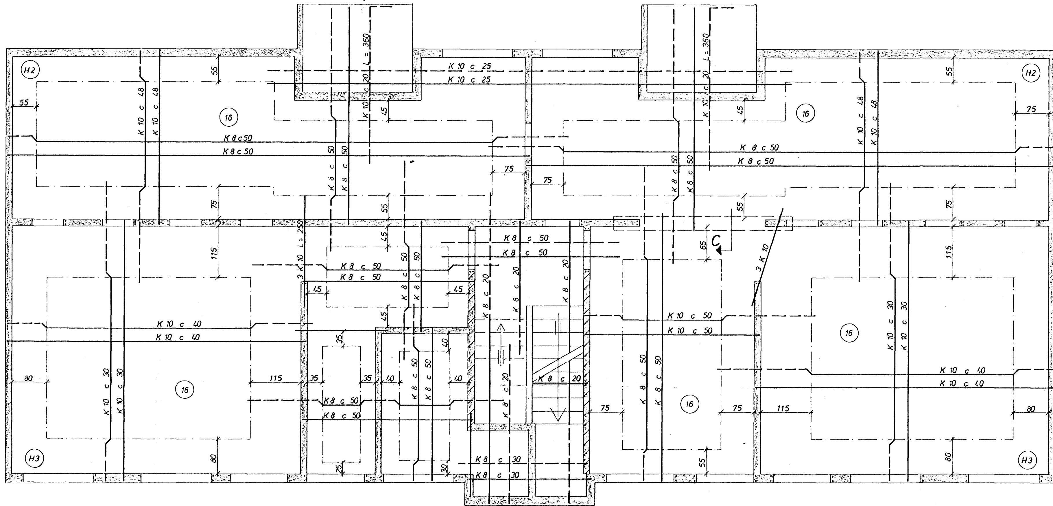
GRUNNMYND 1:50
