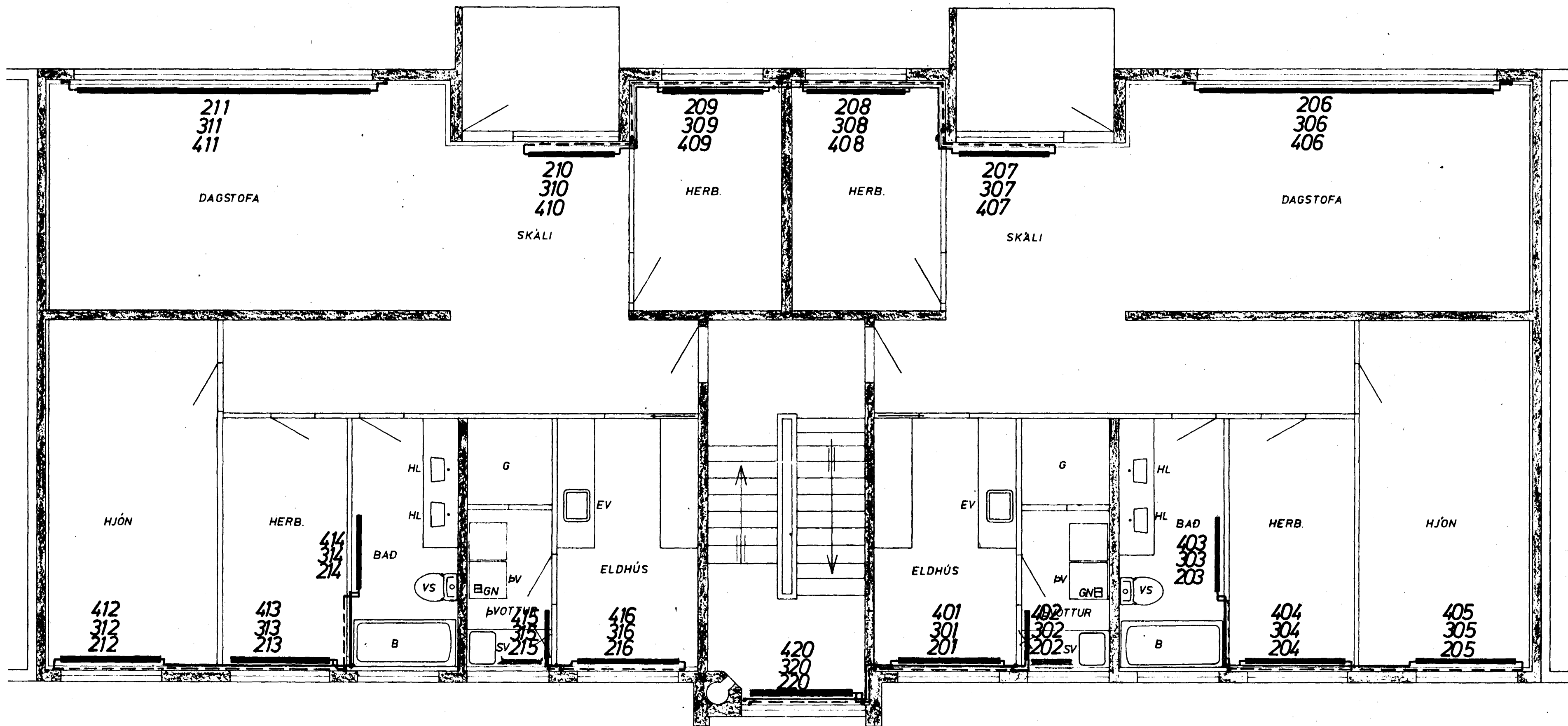
GRUNNMYND 234. HÆÐAR 1:50
