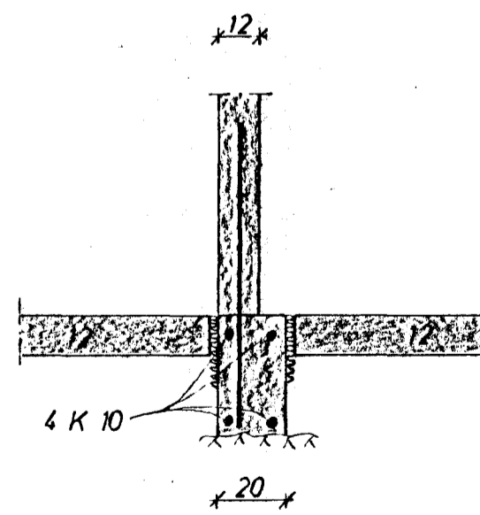
SNID 1 INNVEGG 1:20
