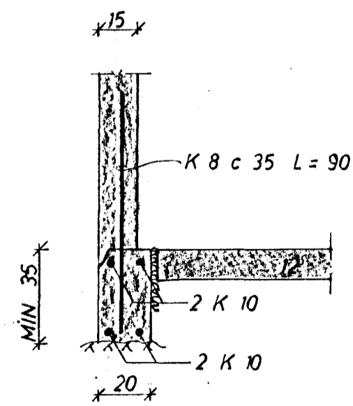
SNID 1 ÚTVEGG 1:20
