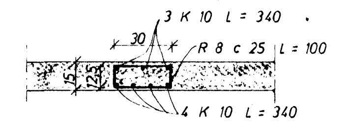
SNID D 1:20
