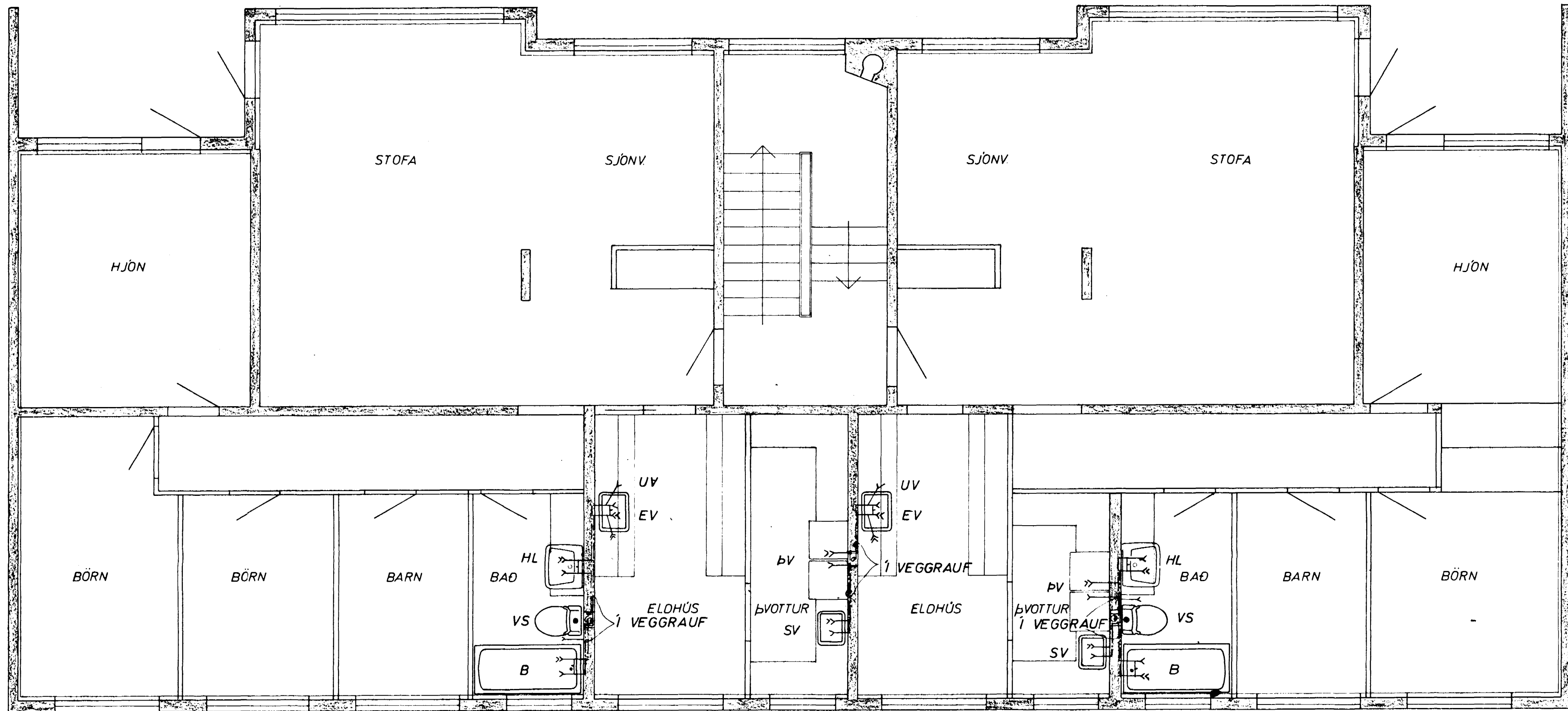
GRUNNMYND 1:50
