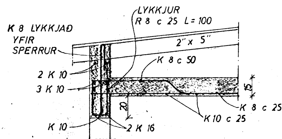
SNID E 1:20
