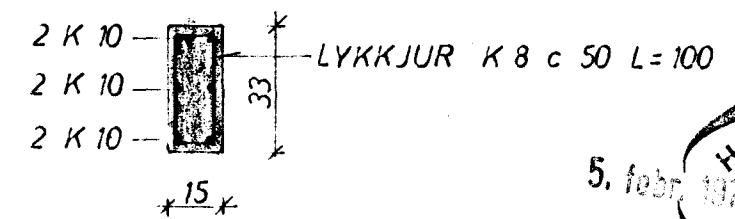
SNID I SÚLUR I STIGAGLUGGA 1:20
