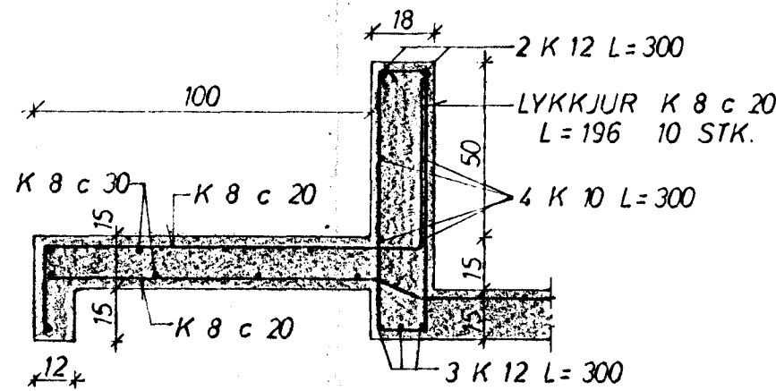
SNID I SKYGGNI
