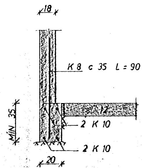
SNID 1 ÚTVEGG 1:20
