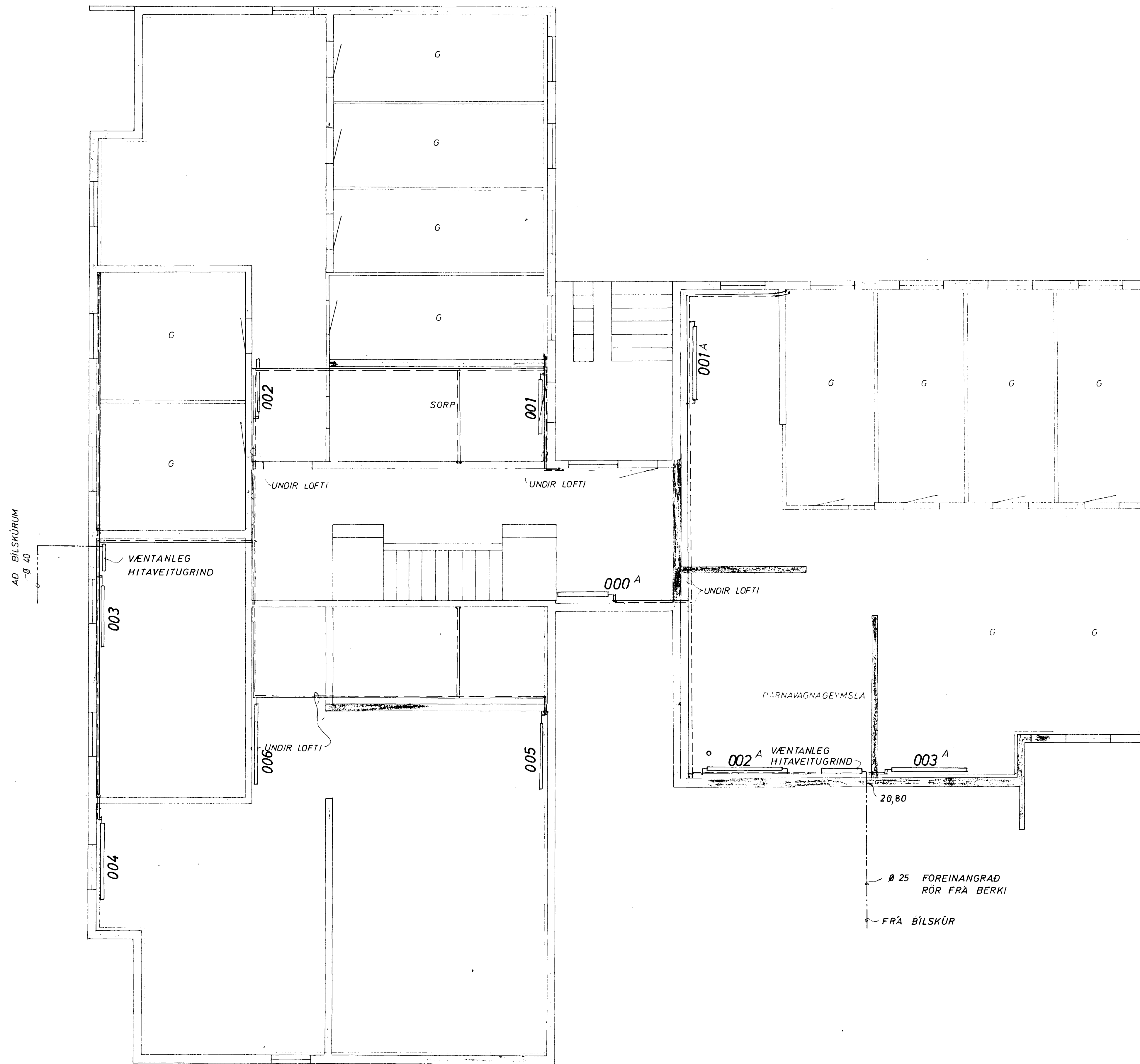
GRUNNMYND KJALLARA 1:50
