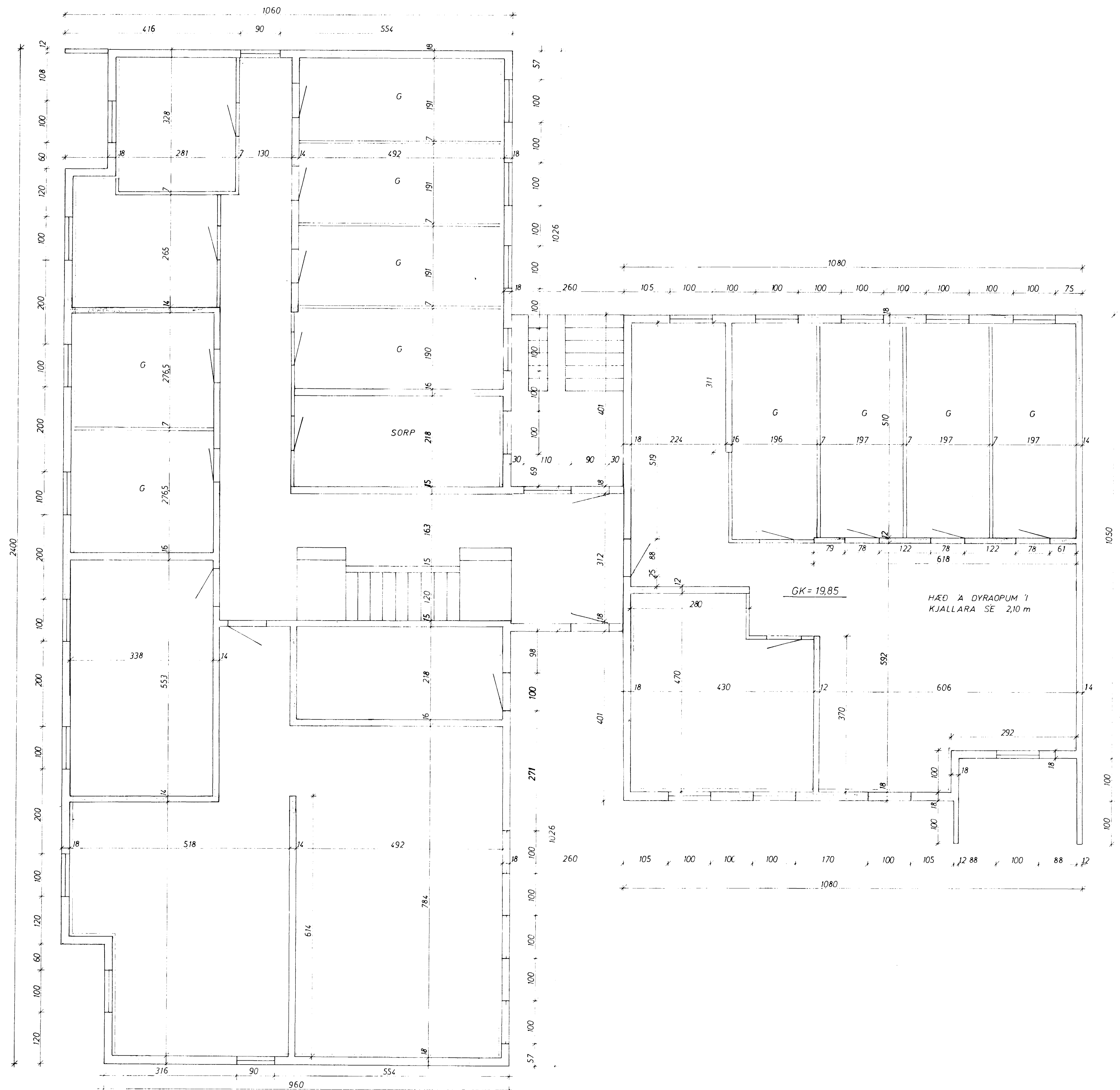
GRUNNMYND KJALLARA 1:50
