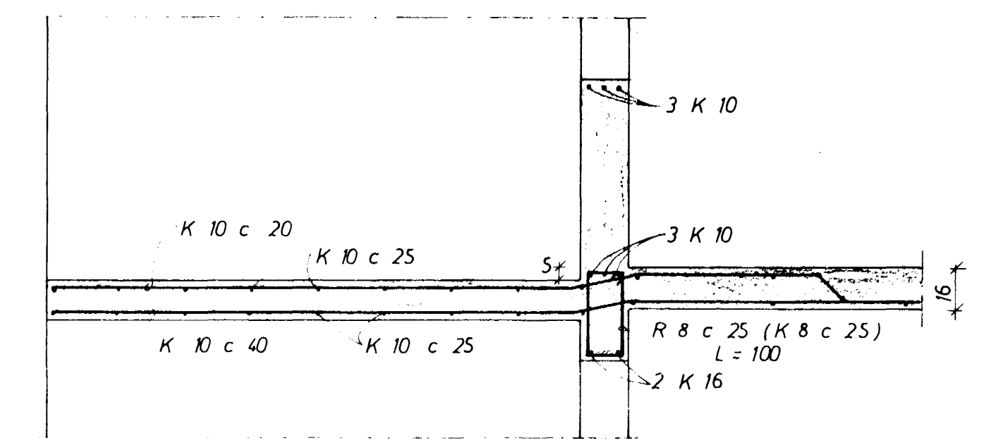
SNID G 1:20
