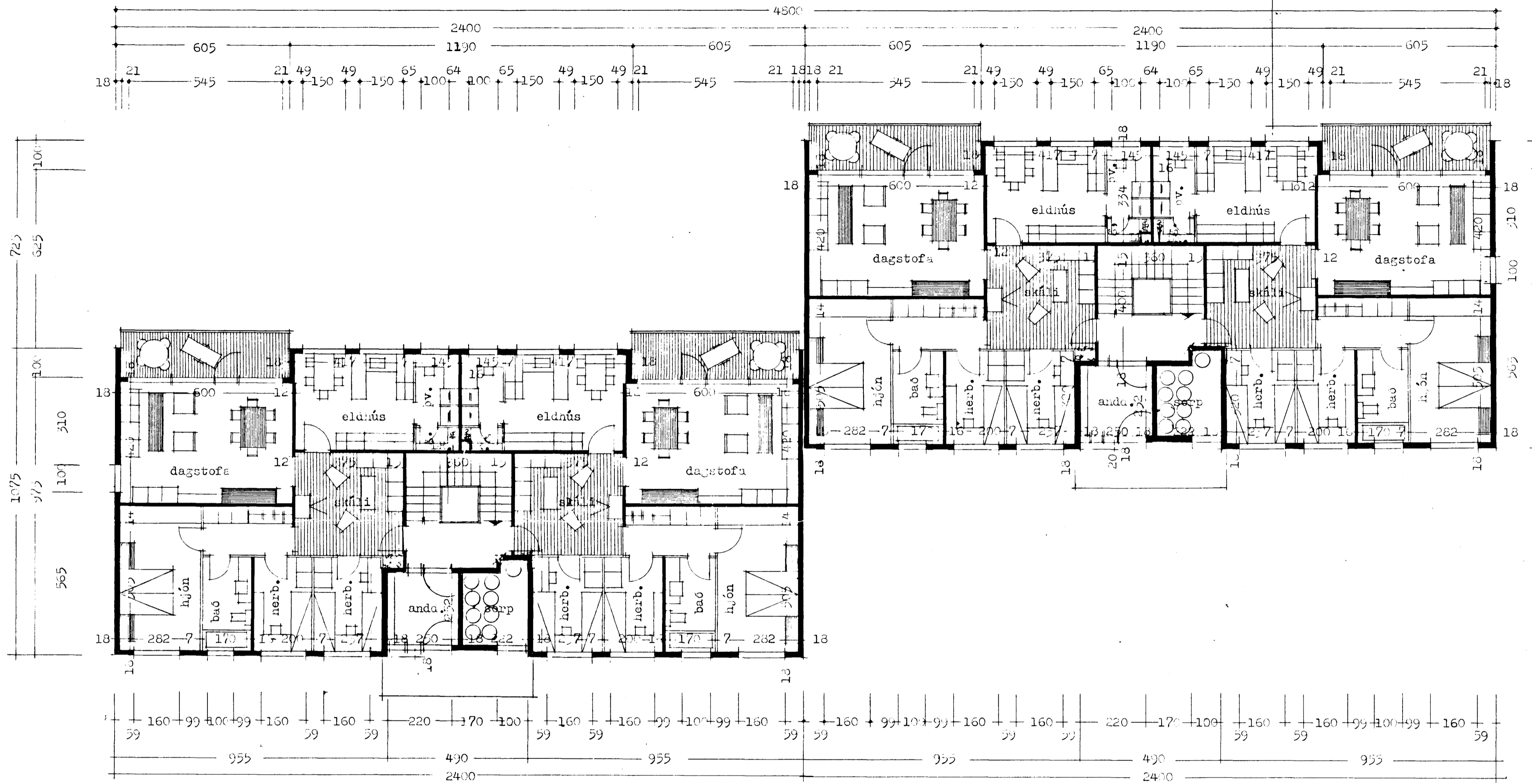
grunnmynd 1. hæð
