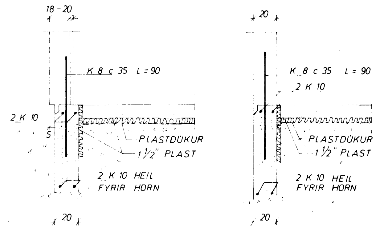
SNID 1 ÚTVEGGI 1:20
