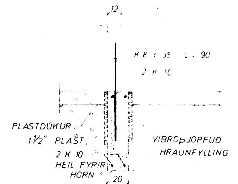
SNID 1 INNVEGGI 1:20
