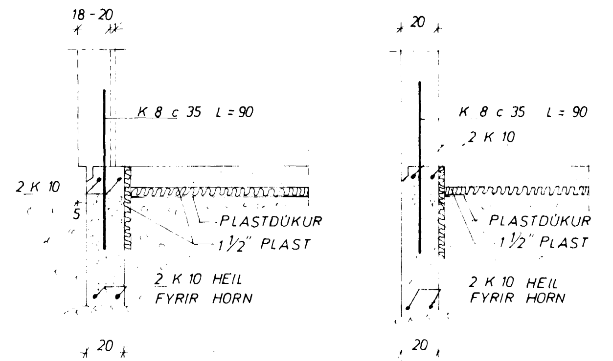
SNID 1 ÚTVEGGI 1:20
