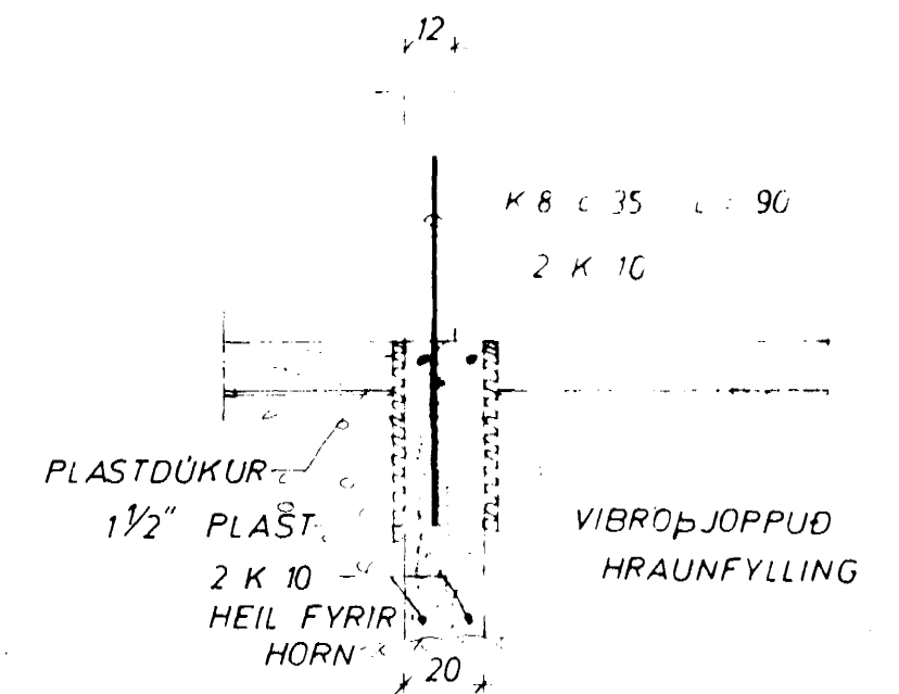
SNID 1 INNVEGG 1:20
