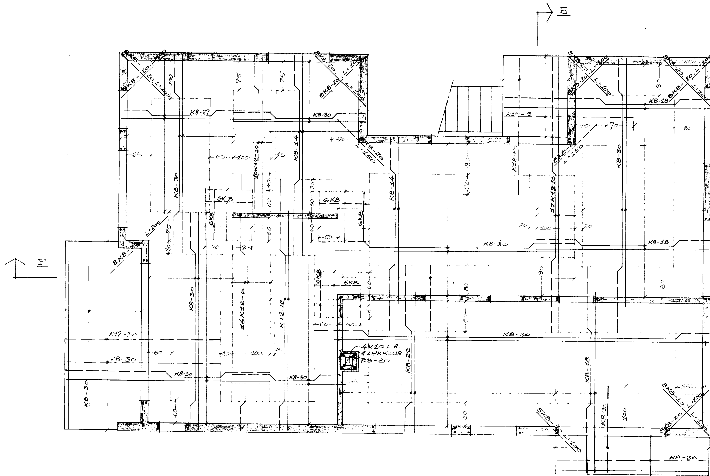
PLATA YFIR 1. HÆÐ, M=1:50
