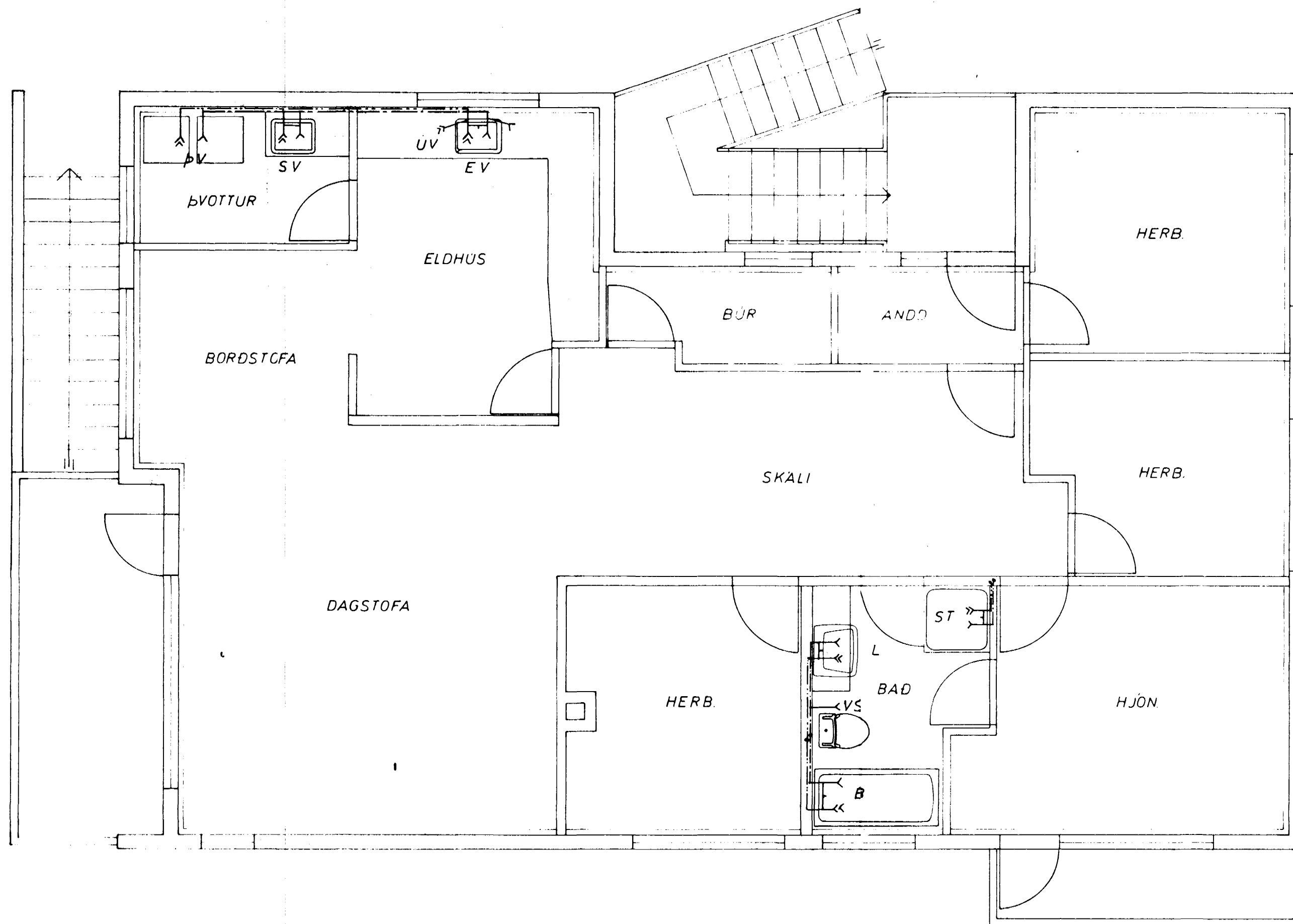
GRUNNMYND 2 HÆÐ 1:50
