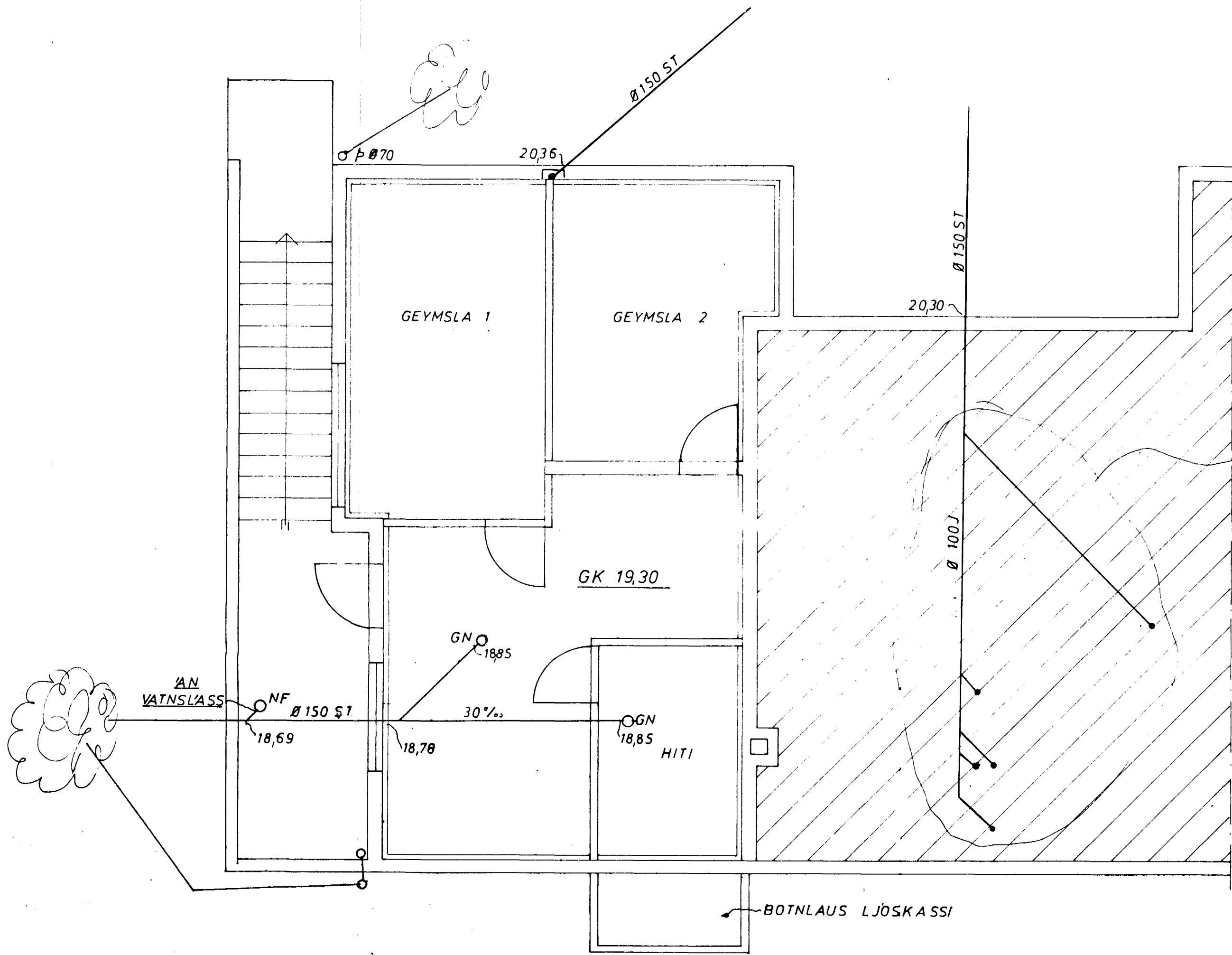
GRUNNMYND KJALLARA 1:50
