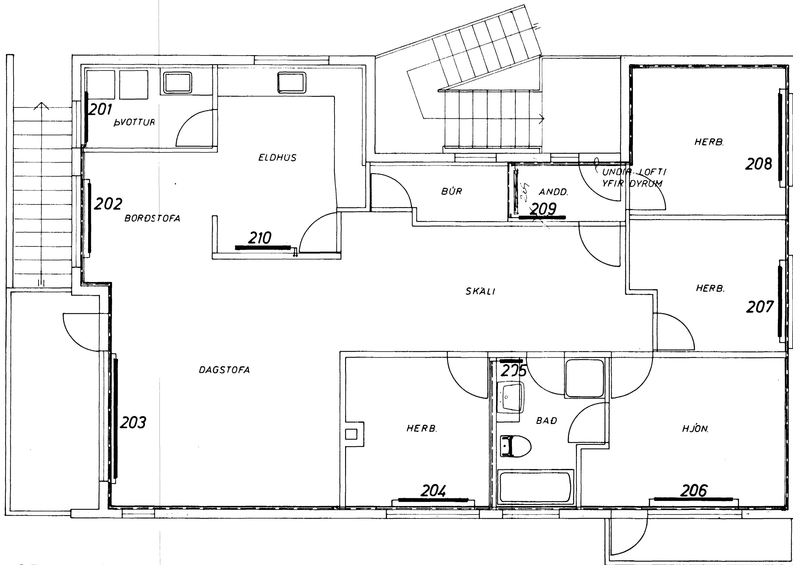
GRUNNMYND 2 HÆÐ 1:50
