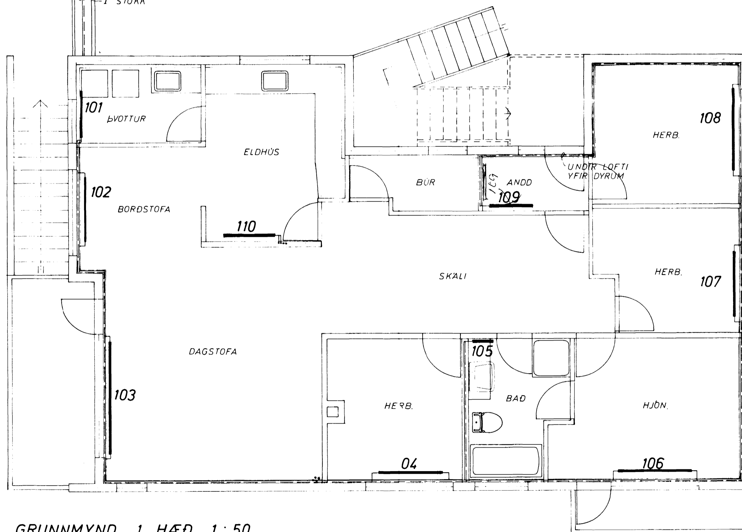
GRUNNMYND 1 HÆÐ 1:50
