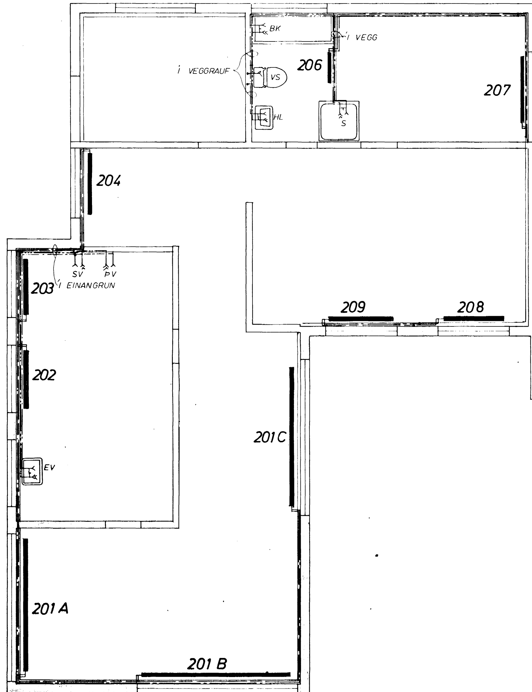
GRUNNMYND 2. HÆÐAR 1:50
